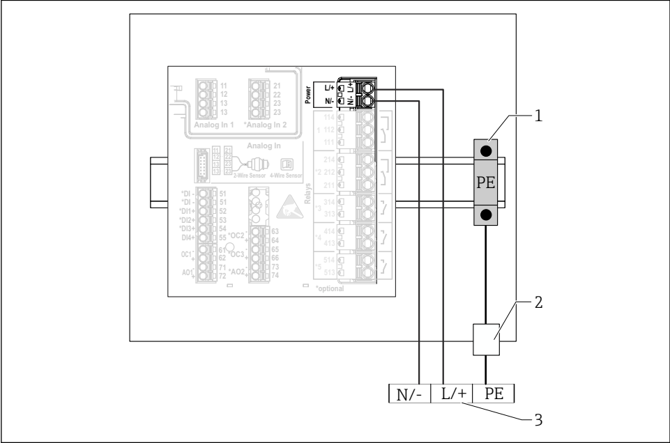
图 16 铝现场型外壳内的电源连接
