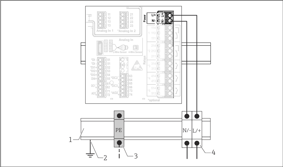
图 17 DIN 导轨式设备上的电源连接
