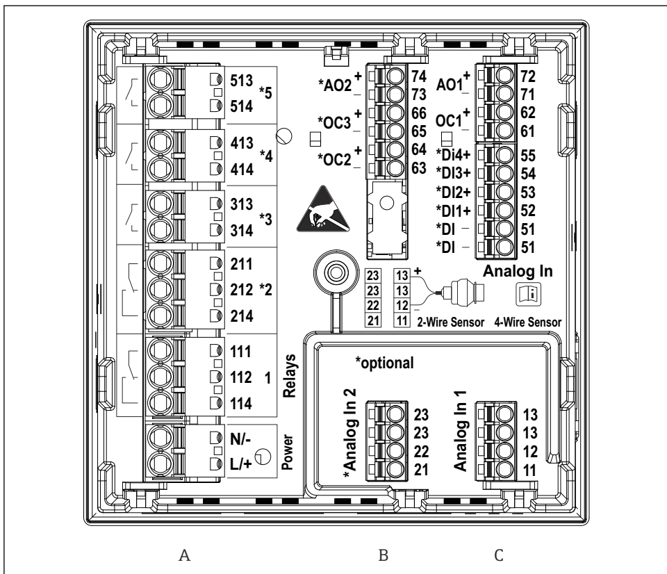
图 9 盘装型设备的接线端子（设备背面）；端子设计：可插拔直推式接线端子
