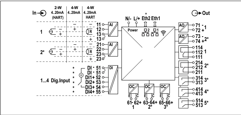
图 13 接线图（标有*的接线端子取决于选型代号）
