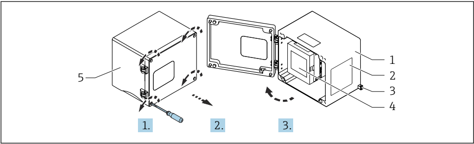
图 7 操作铝现场型外壳的接线腔
