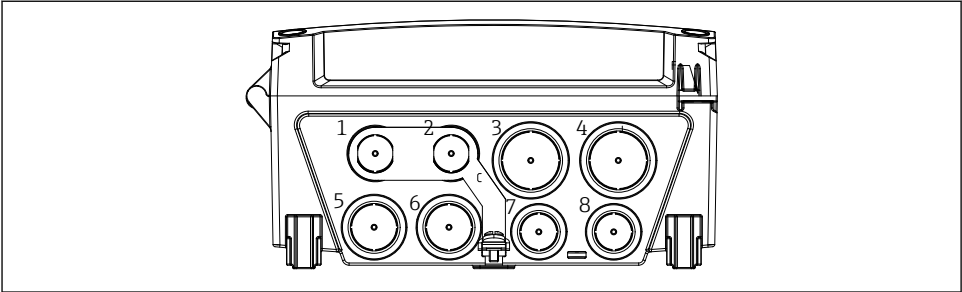
图 6 外壳底部上的预开孔对应下列电缆入口（实例）：
