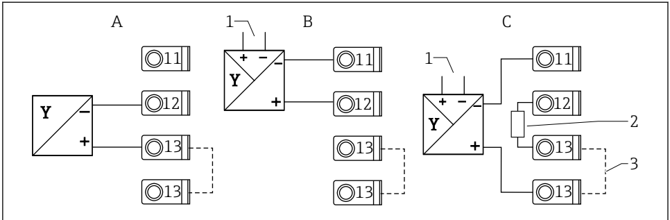
图 14 连接实例：两线制和四线制传感器连接 4...20 mA 电流输入或 HART 通信信号
