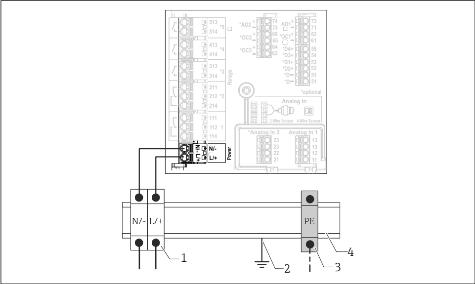
18 盘装型设备上的电源连接
