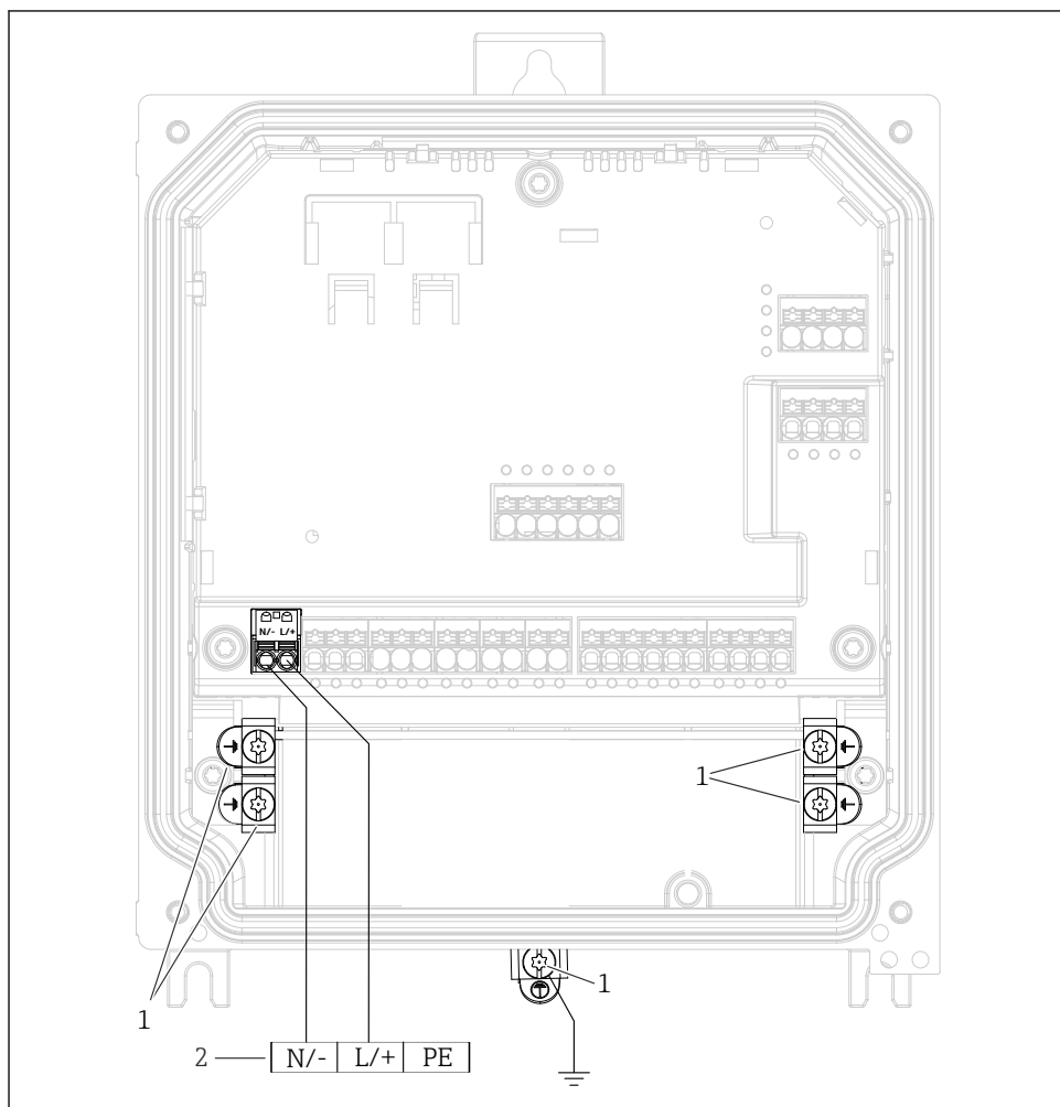
15 聚碳酸酯现场型外壳内的电源连接
