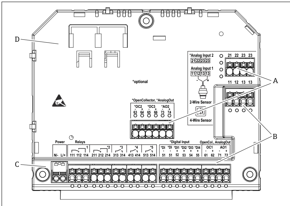
11 聚碳酸酯现场型外壳接线腔中的接线端子；端子设计：直推式接线端子
