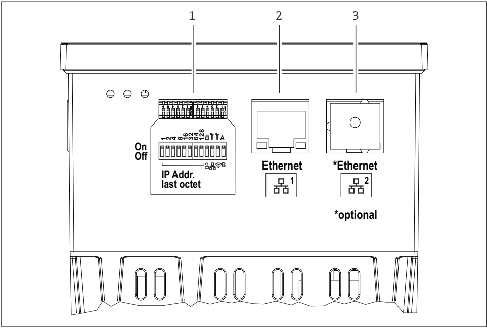
图 10 盘装型设备的连接口（设备底部）
