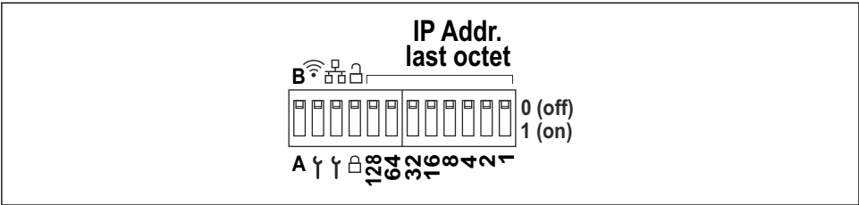
19 DIP 开关（图纸中显示了出厂设置）
