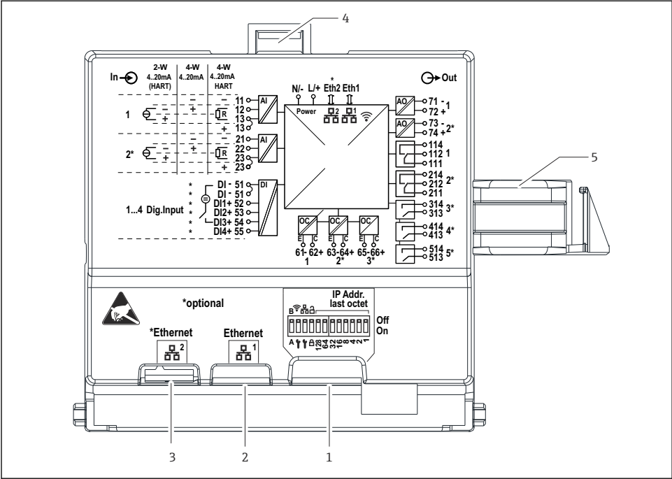
图 12 聚碳酸酯现场型外壳显示单元背面的连接口
