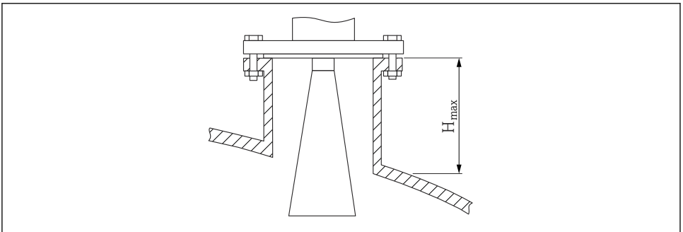
2 Altura do bocal para a antena piramidal (FMR51)
