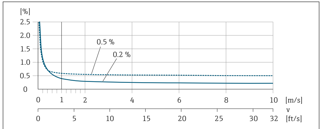
32 Error máximo de medición en % del v. l.
