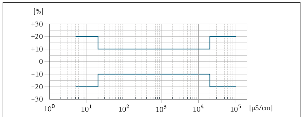
33 Error de medición (estándar)
