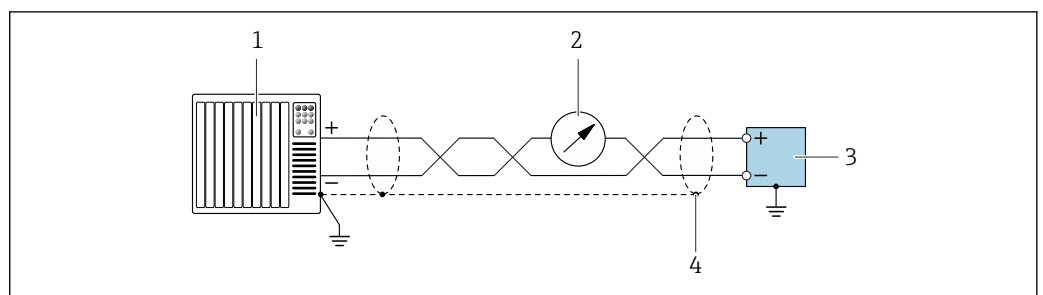
15 Ejemplo de conexión para salida de corriente de 4 ... 20 mA con HART (activa)
