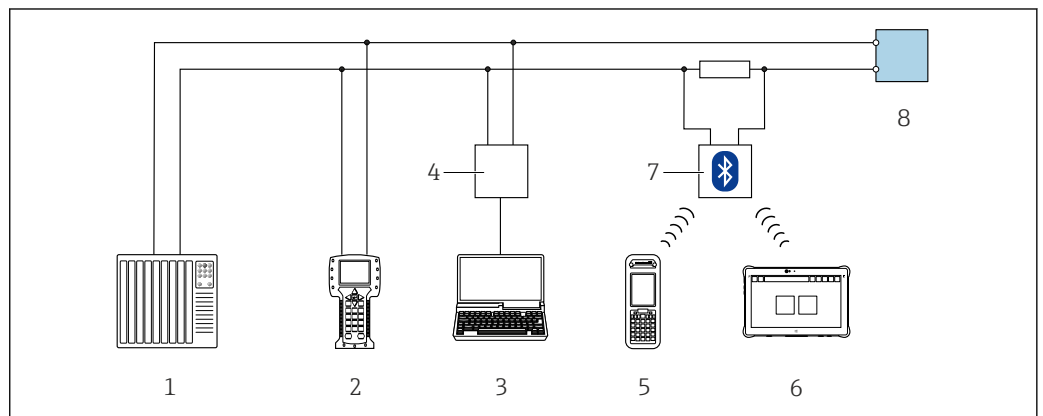
22 Opciones para la configuración a distancia mediante el protocolo HART (activo)
