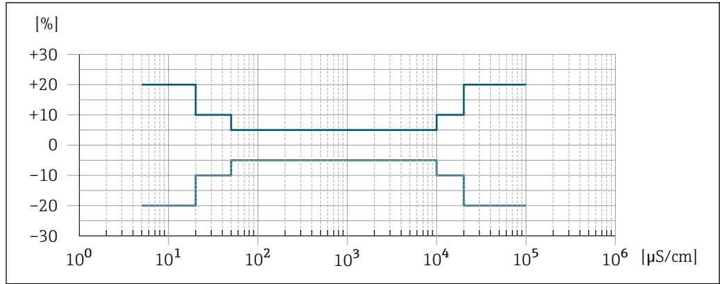
34 Error de medición (opcionalmente: código de pedido para "Medición de la conductividad calibrada", opción CW)
