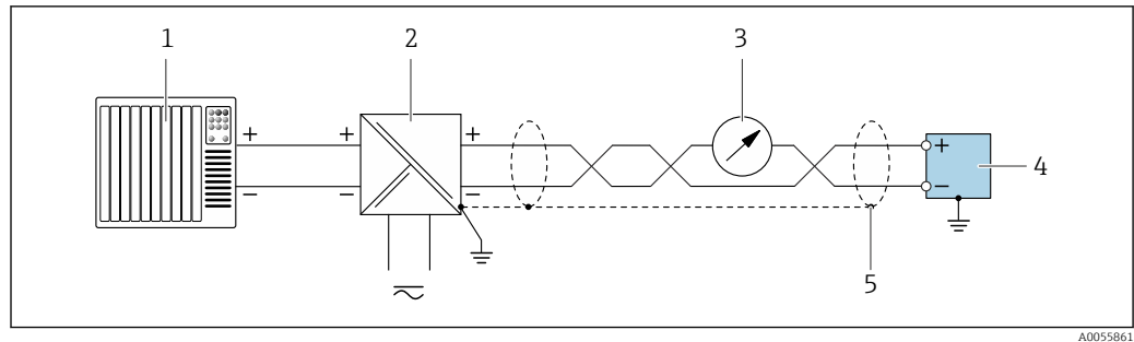
16 Ejemplo de conexión para salida de corriente de 4 ... 20 mA con HART (pasiva)
