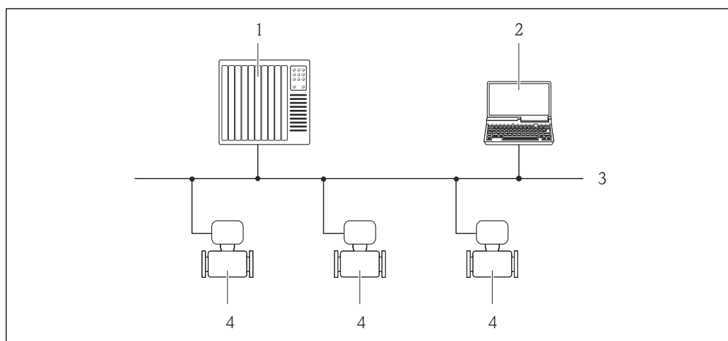
22 Opções para operação remota através da rede PROFIBUS DP
