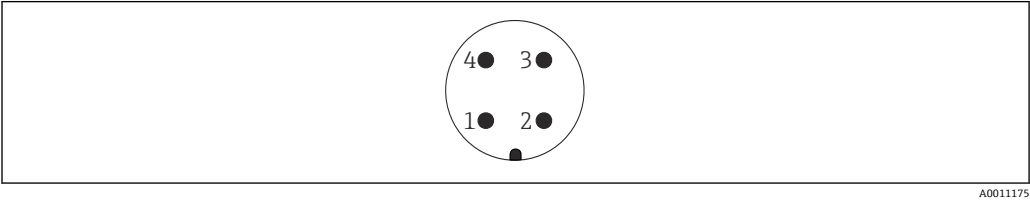
图 4 仪表上的连接插头
