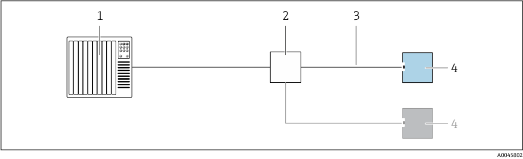
5 接线示例：PROFINET + Ethernet-APL
