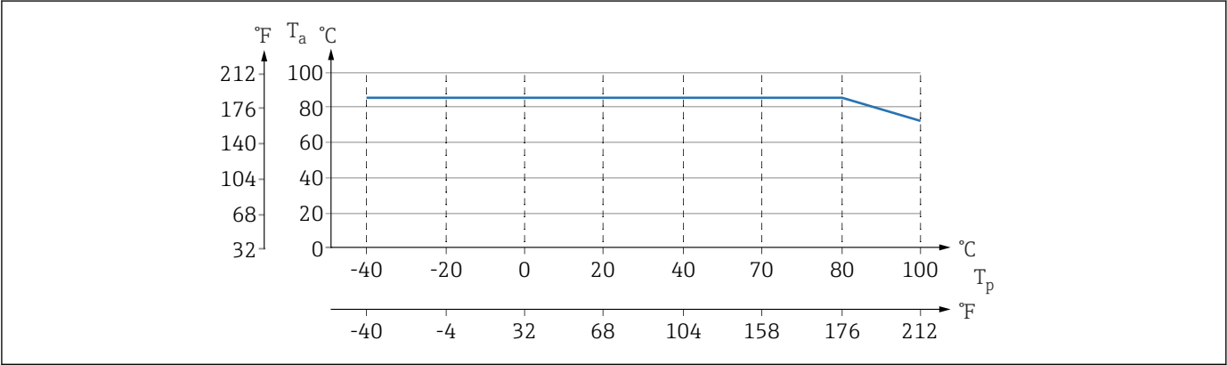
图 6 以上为无保温层竖直安装时的温度范围。 Tp 过程温度 Ta 环境温度
