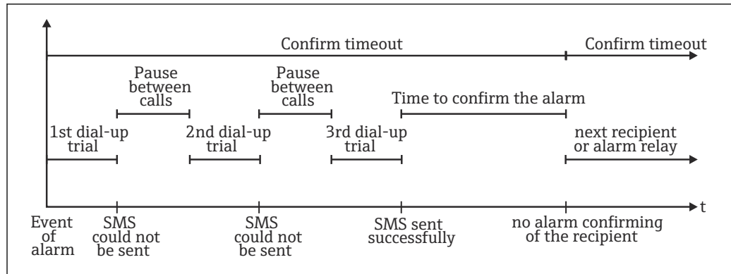
7 Stapvolgorde in geval van een alarm: zenden en bevestigen van telealarms via SMS
