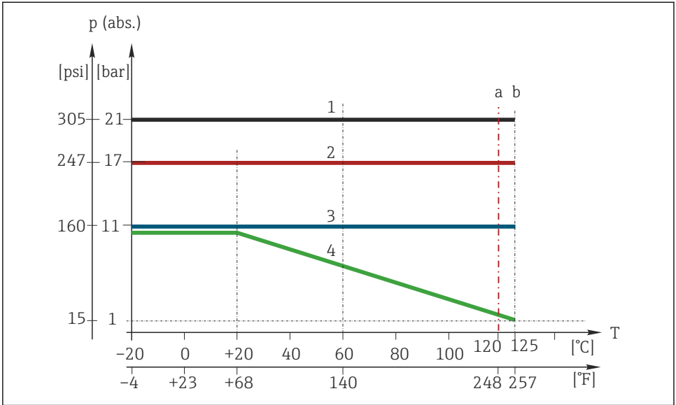
图 10 温压曲线
