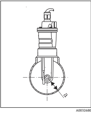
图 5 CLS54 的安装示意图
