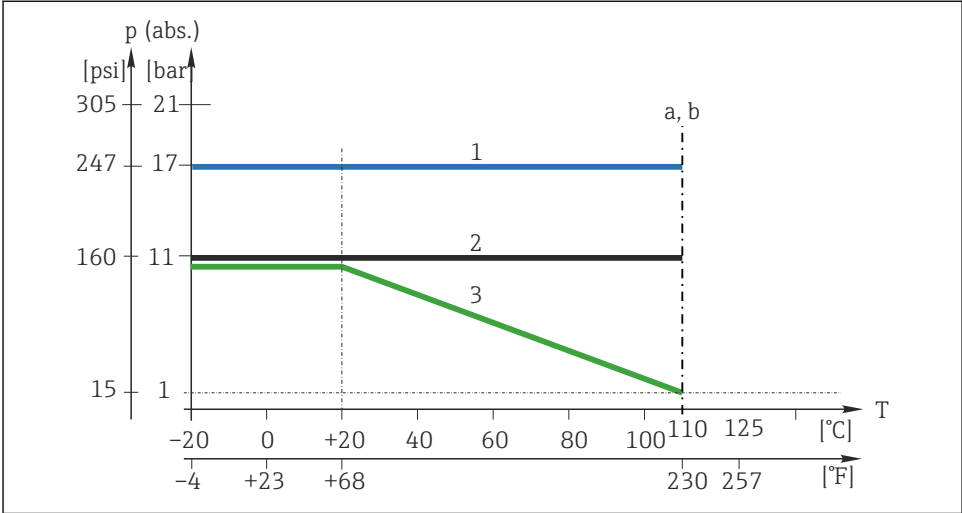
11 温压曲线
