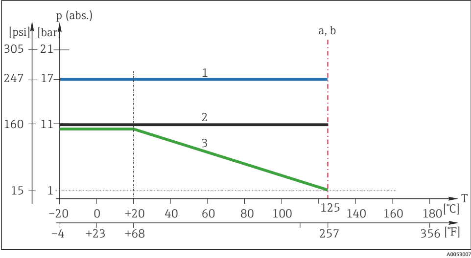
13 温压曲线
