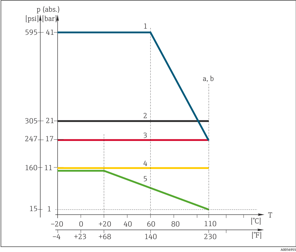
9 温压曲线
