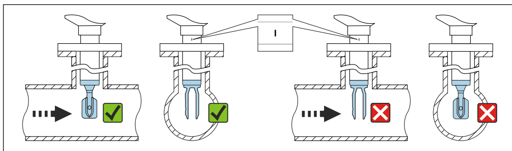
13 Einbau in Rohrleitungen (Gabelstellung und Markierung berücksichtigen)
