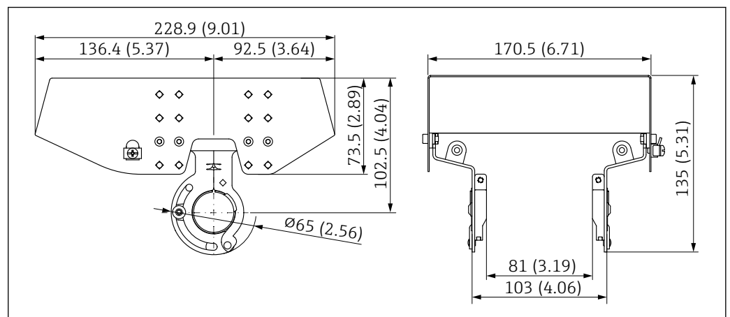
30 Wetterschutzhaube für Zweikammergehäuse. Maßeinheit mm (in)
