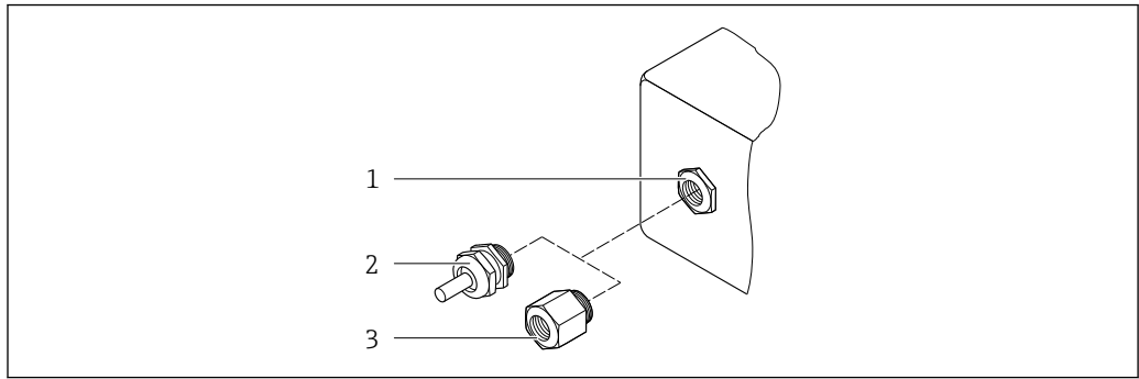
45 Entradas de cable/prensaestopas posibles
