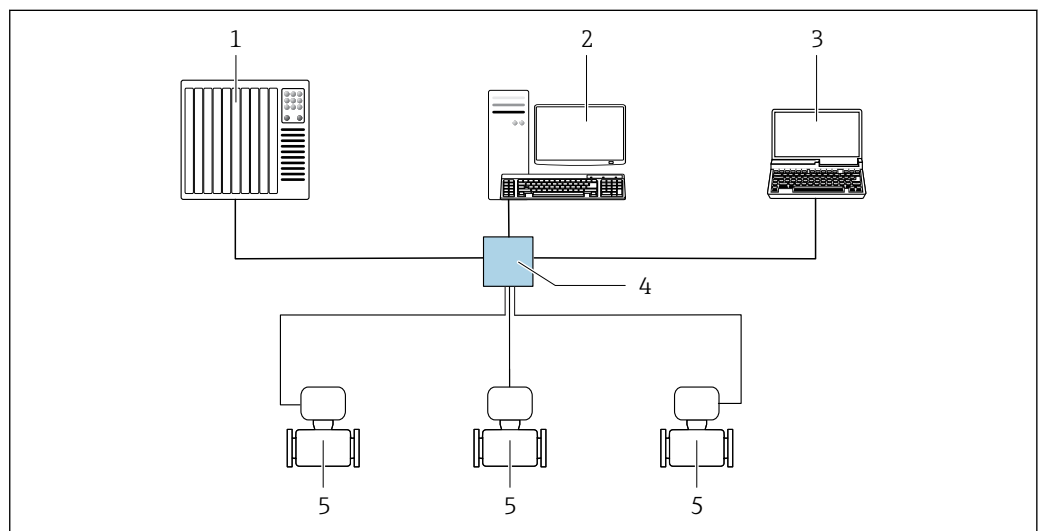
23 Opciones para la configuración a distancia mediante red Ethernet/IP: topología en estrella
