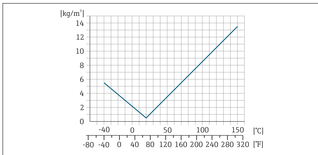
34 Калибровка по плотности на месте эксплуатации, в примере при +20 °C (+68 °F)
