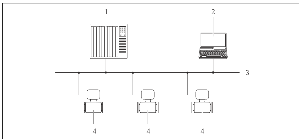
24 Варианты дистанционного управления через сеть PROFIBUS DP
