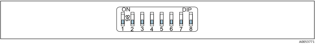
9 软件地址设定示意图；开关 8 拨至“OFF”位置，进入操作菜单设置地址
