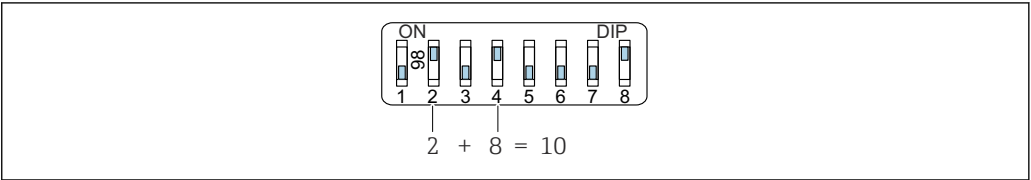
10 硬件地址设定示意图；开关 8 拨至“ON”位置，使用开关 1...7 设置设备地址
