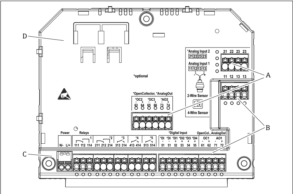
45 Terminais no compartimento de terminais do invólucro de campo de policarbonato; design do terminal: terminais push-in
