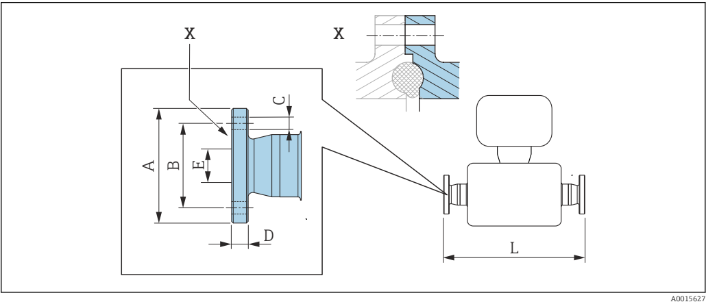
32 Détail X : Raccord process asymétrique, la partie bleue fait partie de la livraison.
