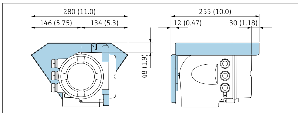
43 Capot de protection climatique pour Proline 500 – unité mm (in)
