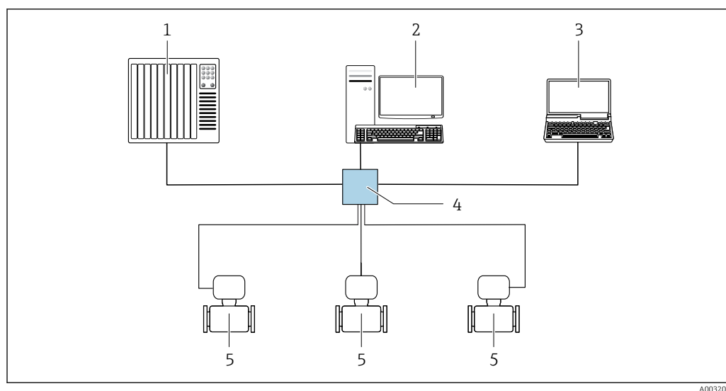
56 Options pour la configuration à distance via le réseau EtherNet/IP : topologie en étoile
