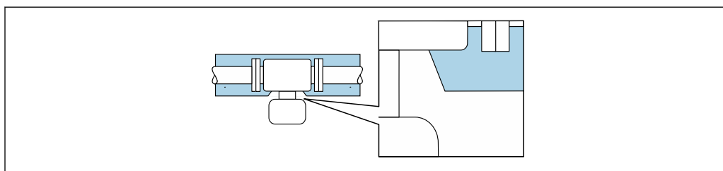
31 Isolation thermique avec tube prolongateur exposé
