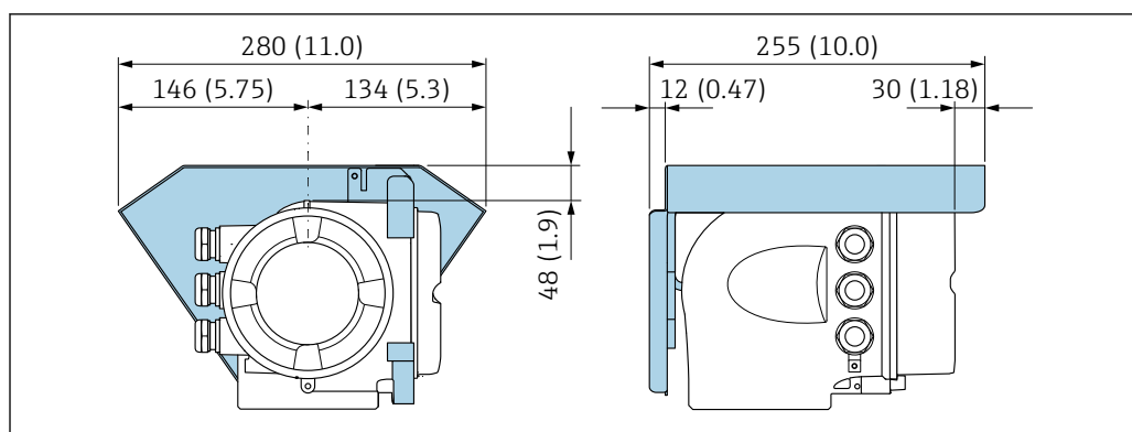
36 Capot de protection climatique pour Proline 500 – unité mm (in)
