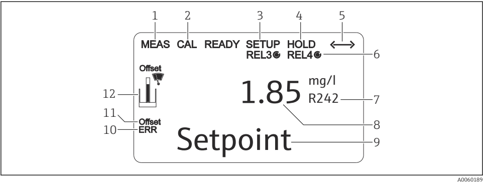
15 Afișaj transmițător LC
