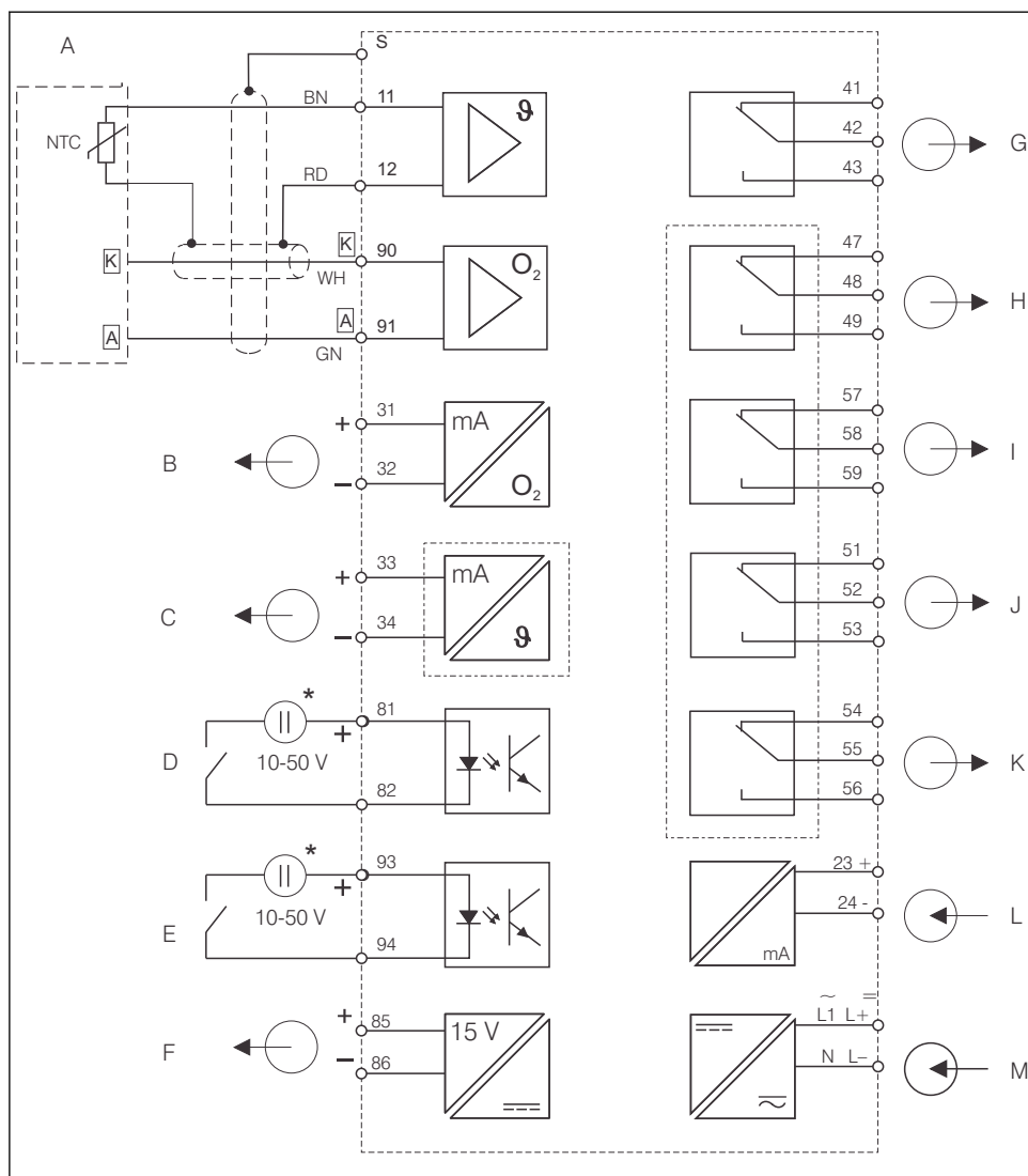
7 Conexiunea electrică a transmițătorului, versiunea DX sau DS
