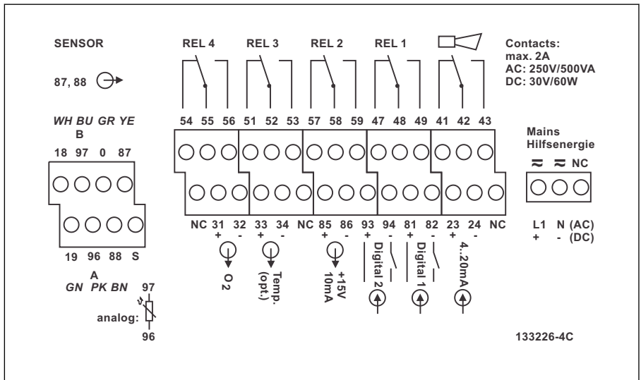
11 Etichetă compartiment de conexiuni Liquisys M, versiunea WX/WS
