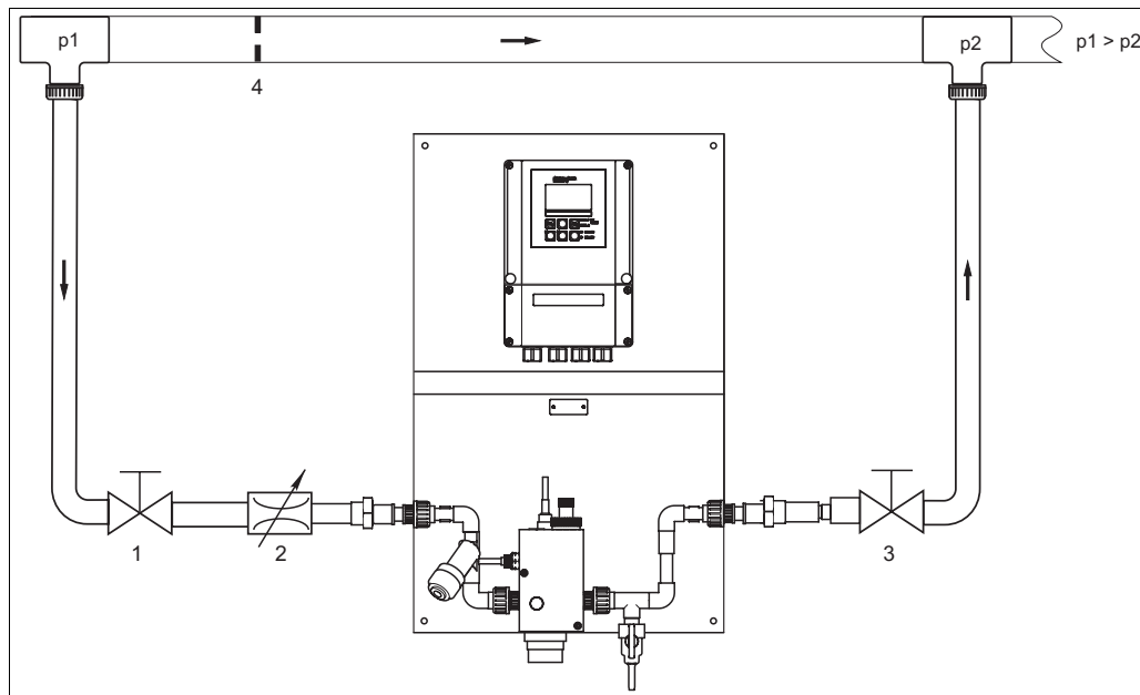
Exemple de raccordement avec bypass et diaphragme dans la conduite principale
