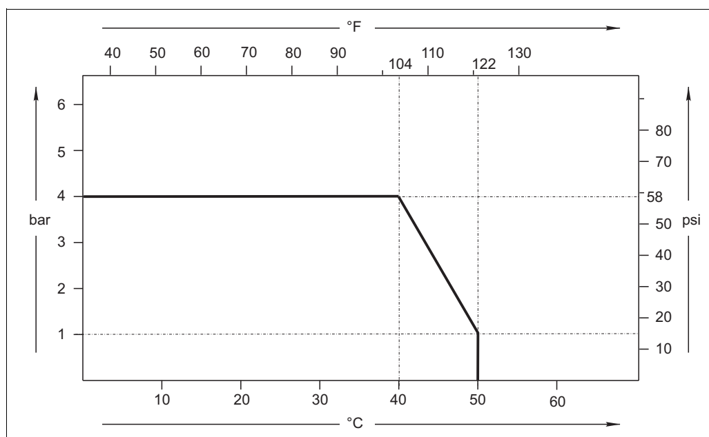
Fig. 2 : Diagramme de pression et de température
