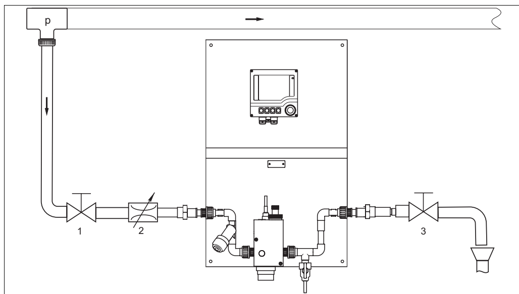
Exemple de raccordement avec écoulement ouvert
