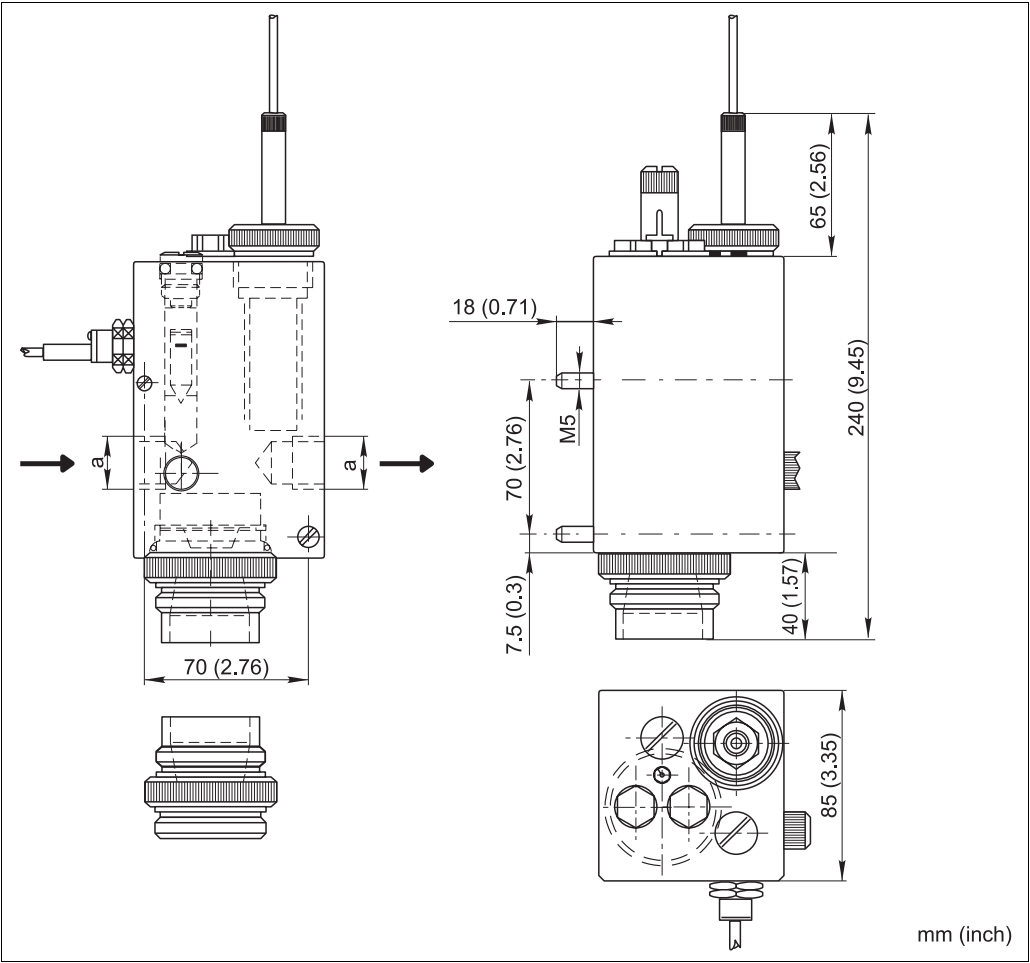
Fig. 3 : Dimensions a En fonction de la version : G1/2, NPT 1/2" ou NPT 1/4"
