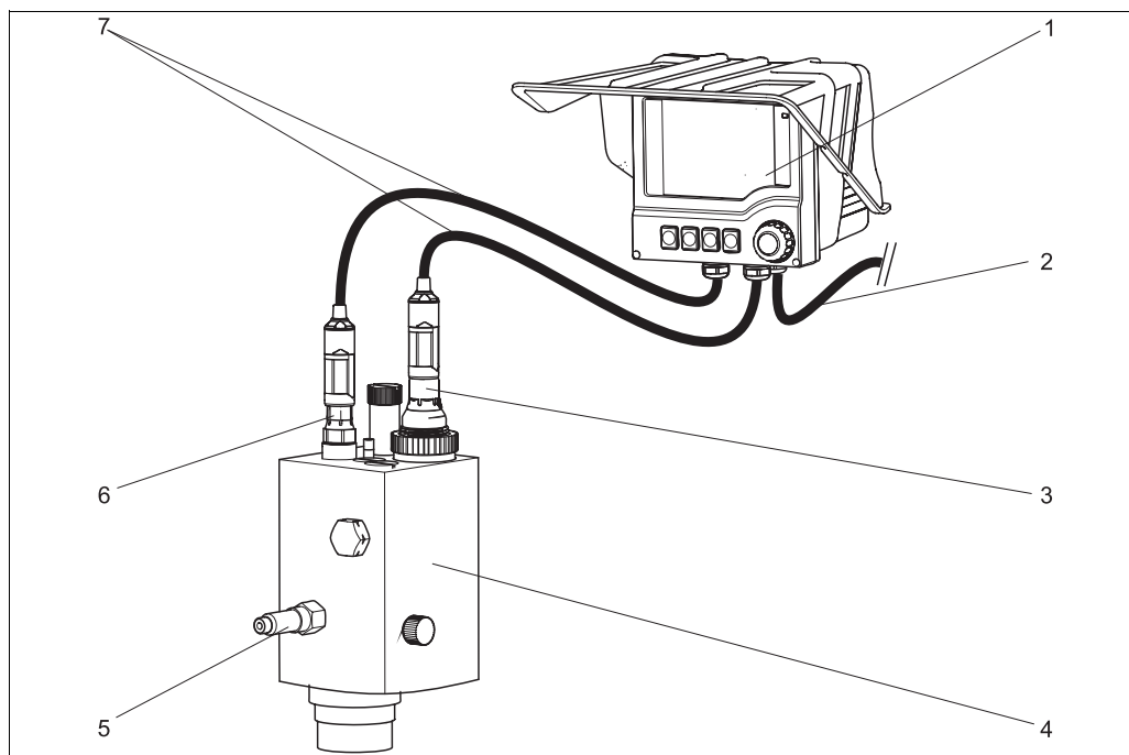
Fig. 1 : Exemple d'ensemble de mesure
