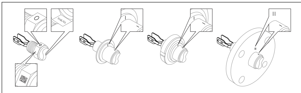
图 13 参照标记水平安装在罐体中的音叉位置
