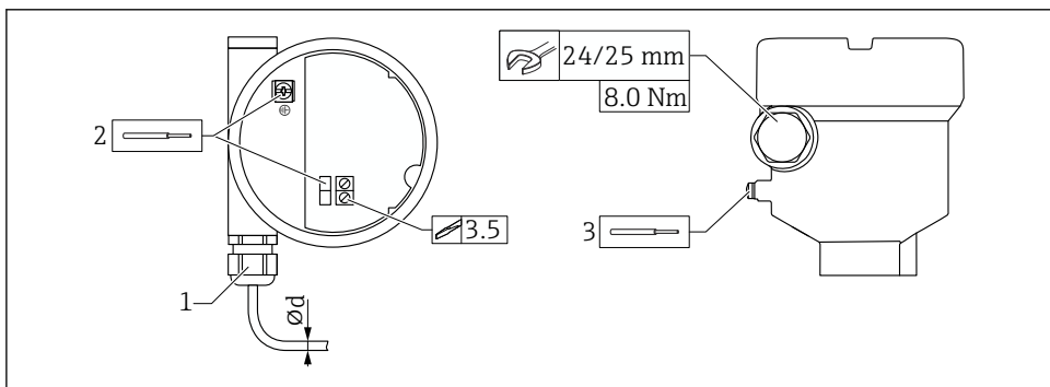
图 20 实例：接头（带电缆入口）和电子插件（带接线端子）
