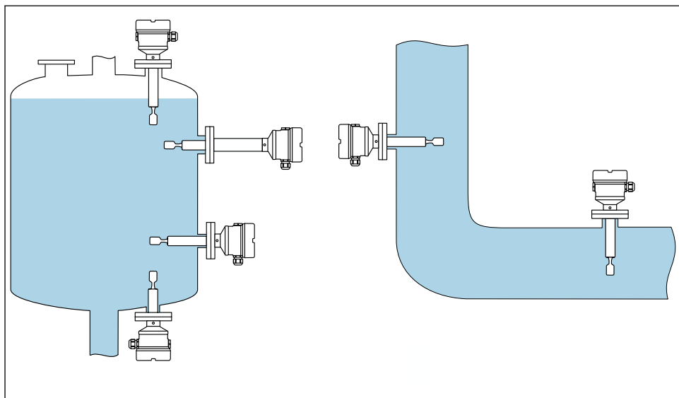
图 4 安装实例：安装在容器、罐体或管道中
