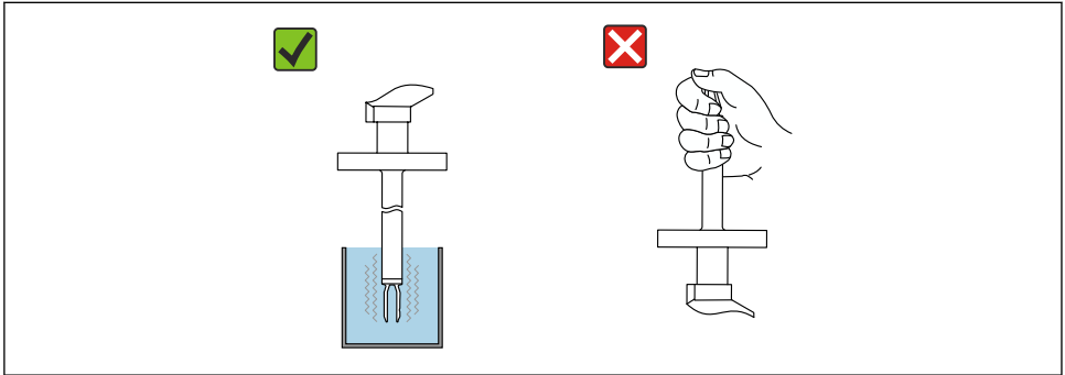
图 22 音叉的功能测试
