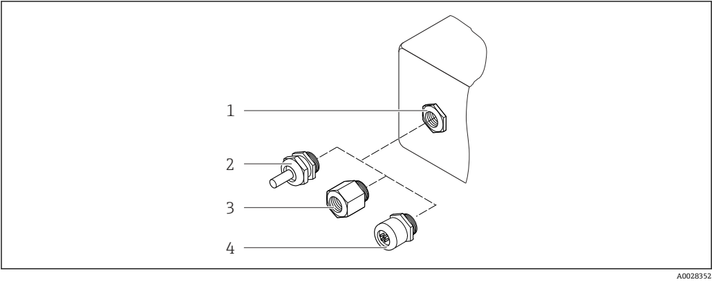
图 37 允许的电缆入口/缆塞 1 M20 × 1.5 内螺纹 2 M20 × 1.5 缆塞 3 转接头，适用 G ½"或 NPT ½"内螺纹电缆入口 4 设备插头
