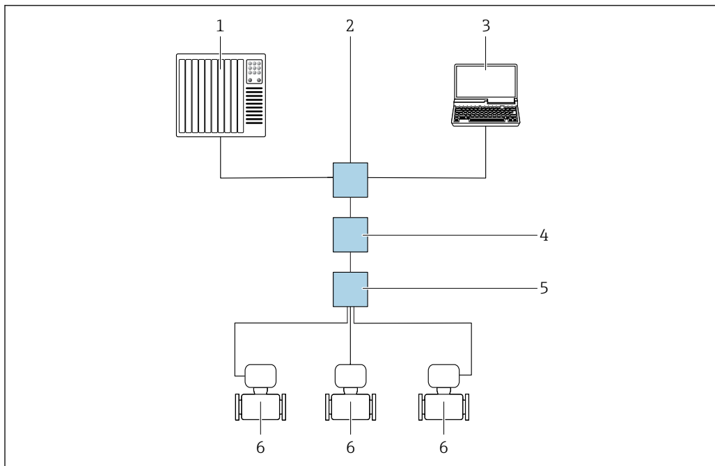
图 46 通过 Modbus TCP + Ethernet-APL 通信进行远程操作（有源信号）
