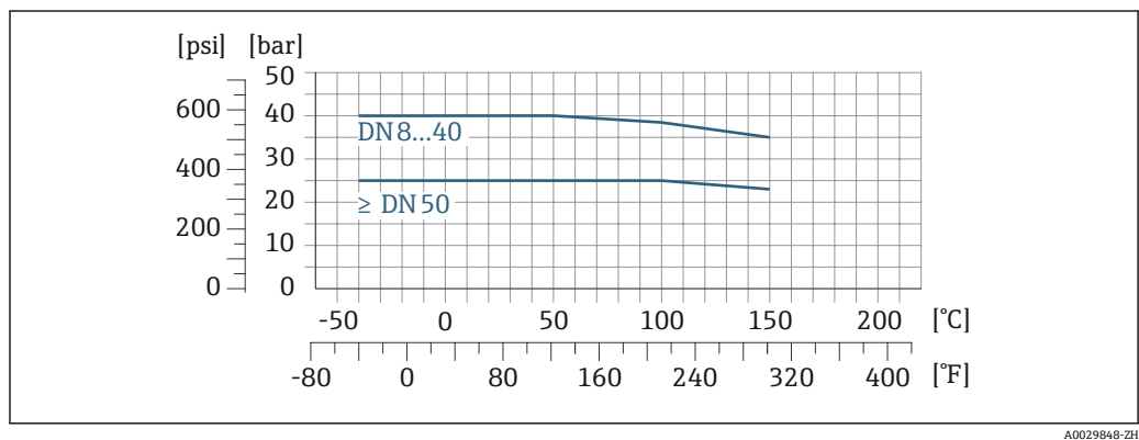
图 22 连接部件材质: 1.4404 (316/316L)
