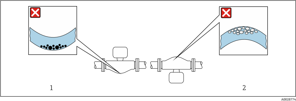
图 15 弯测量管传感器的安装方向
