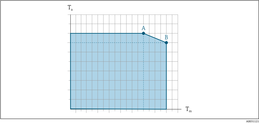
图 17 示例图，具体数值见下表。 T a 环境温度 T m 介质温度 A 介质温度 T m 越高 (T a max = 60 °C (140 °F) 时)，所需的环境温度 T a 越低 B 传感器最高允许介质温度 T m 对应的最高允许环境温度 T a
