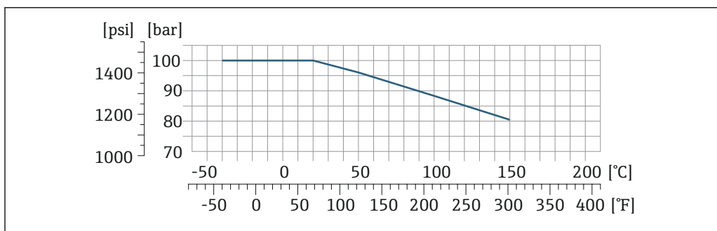
图 26 连接部件材质: 1.4404 (316/316L)
