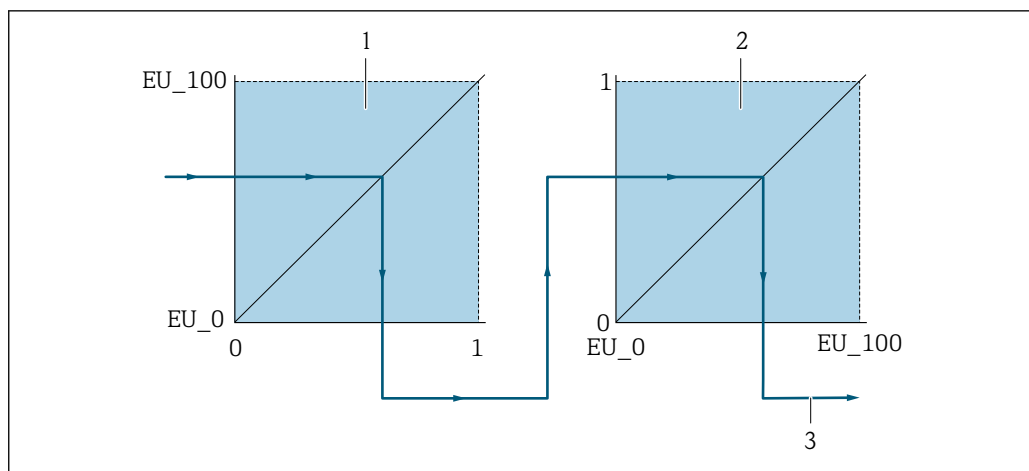
18 Escalado del valor medido en el bloque de entradas analógicas
