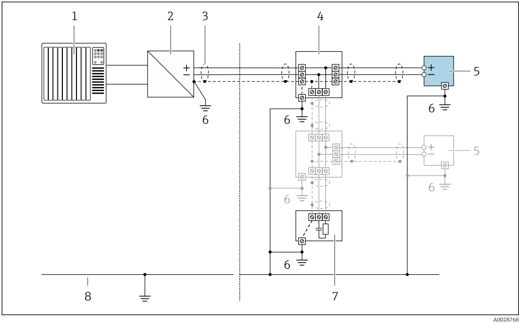
8 Ejemplo de conexión para FOUNDATION Fieldbus
