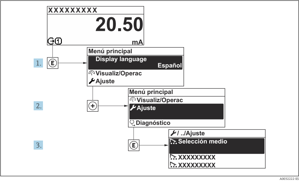
16 Acceso al Menú "Ajuste" usando el ejemplo del indicador local
