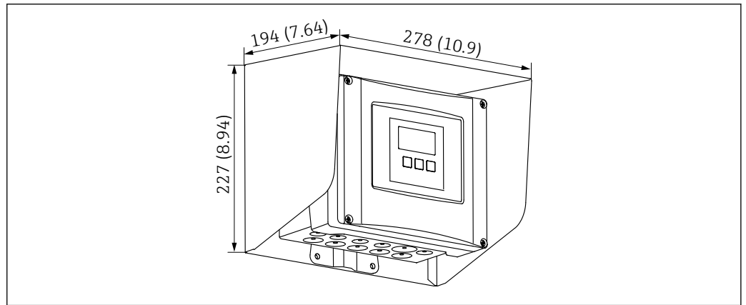
■ 61 Tettuccio di protezione dalle intemperie per custodia da campo in policarbonato. Unità di misura mm (in)
