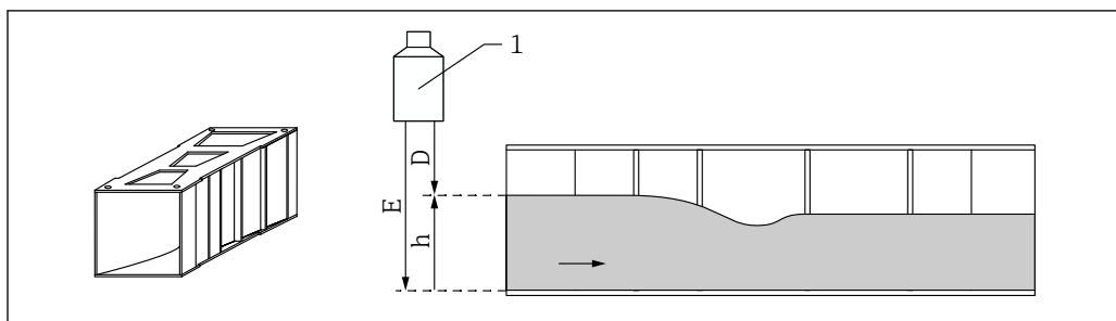
46 Calibrazione di vuoto per canale aperto
