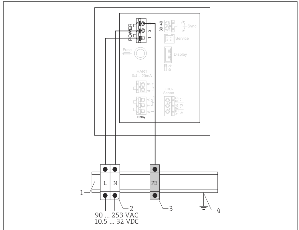
24 Collegamento dell'alimentazione nella custodia per guida DIN
