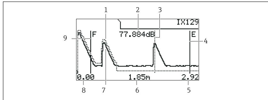
60 Curva di inviluppo sul display locale
