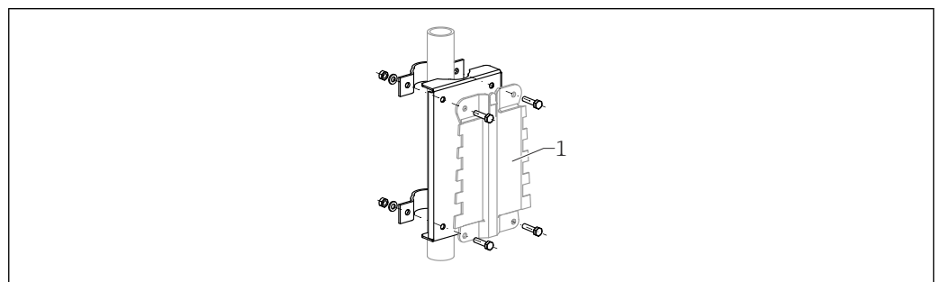
■ 62 Piastra di montaggio della custodia da campo in policarbonato
