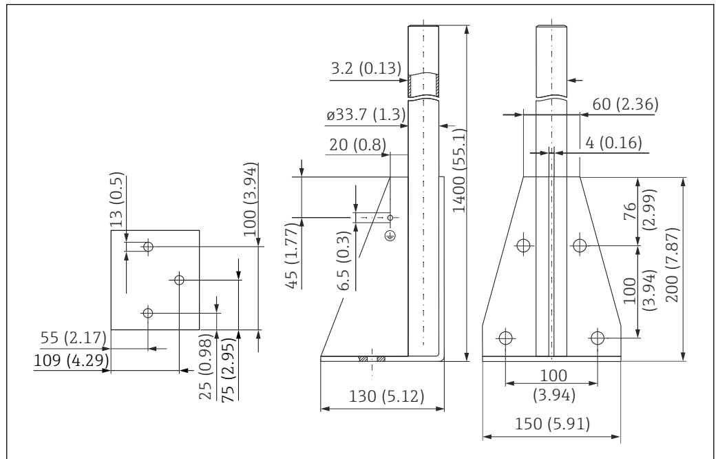
64 Dimensioni. Unità di misura mm (in)
