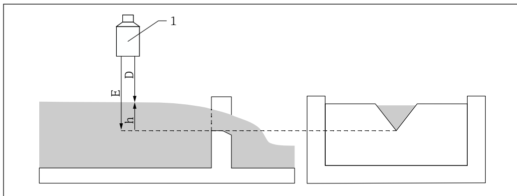
47 Calibrazione di vuoto per stramazzi
