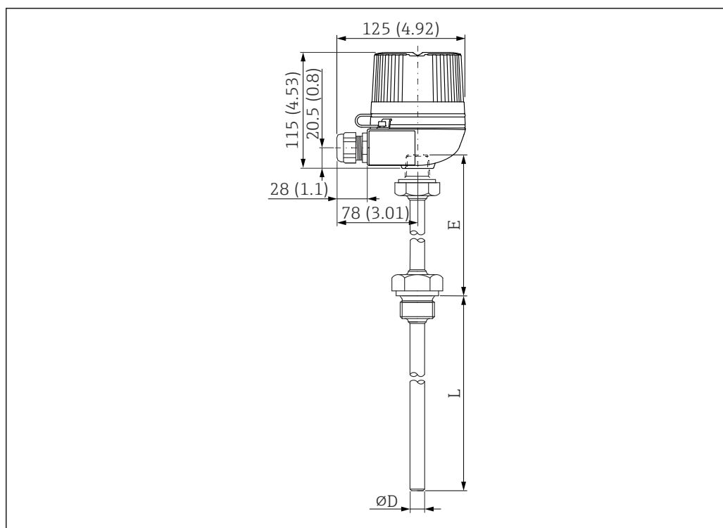
66 Struttura di Omnigrad S TR61; dimensioni: mm (in)
