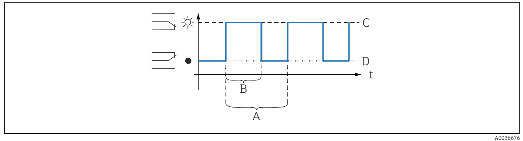
■ 58 Configurazione di un relè a impulsi temporizzati
