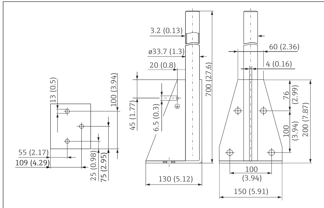
63 Dimensioni. Unità di misura mm (in)
