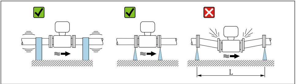
図 6 機器振動の防止対策 (L > 10 m (33 ft))
