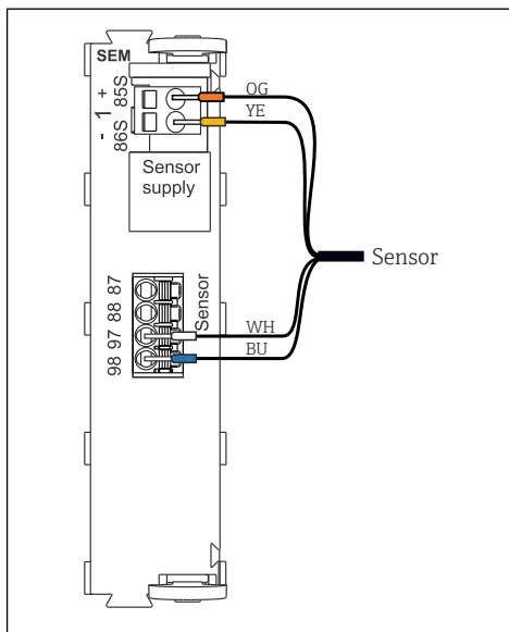
31 Spektrometertilkobling til SEM/modul
