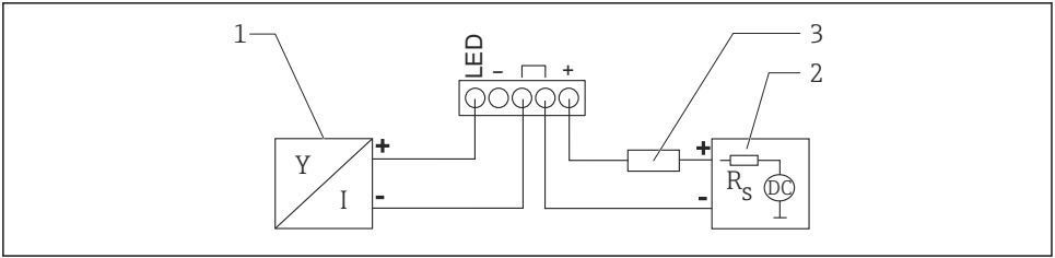
12 Işıklı RIA15 proses indikatörlü HART cihazının fonksiyon şeması
