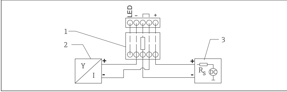
■ 13 HART cihazının fonksiyon şeması, ışısız RIA15, HART iletişim direnç modülü
