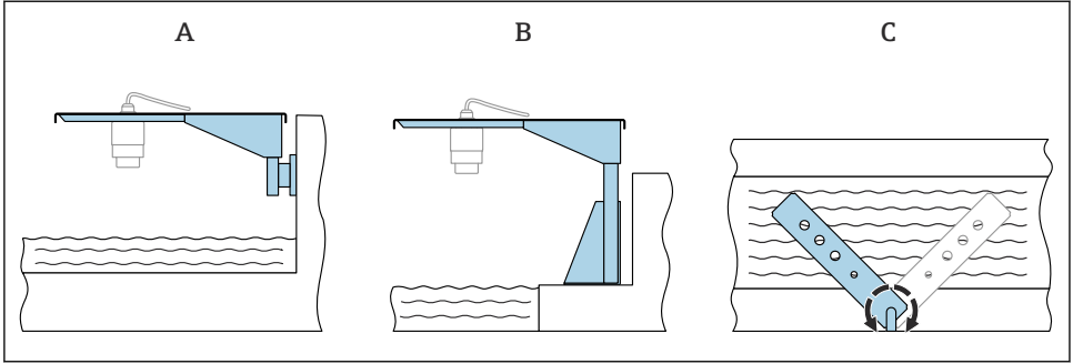
7 Destek kurulumu, eksenli
