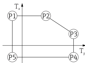
14 Пластмассовый корпус; рабочая температура -20 до +150 °C ( -4 до +302 °F)
