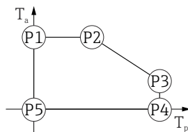
13 Пластиковый корпус; рабочая температура 0 до +200 °C ( +32 до +392 °F) для сертификата CSA C/US
