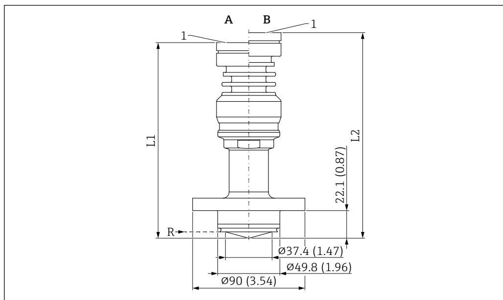
54 Размеры антенны с покрытием, монтаж заподлицо, ПЭЭК, 40 мм (1,5 дюйм), NEUMO BioControl D50. Единица измерения мм (дюйм)
