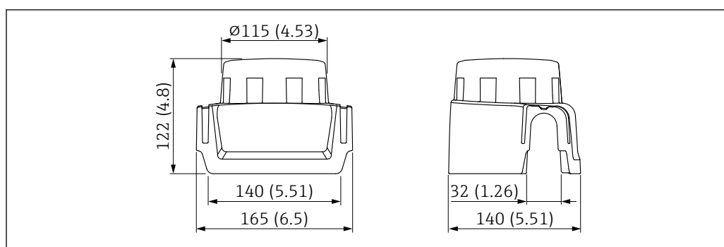
66 Размеры защитного козырька от погодных явлений, пластмасса, XW111. Единица измерения мм (дюйм)
