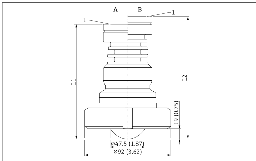
47 Размеры плакированной материалом PTFE антенны, монтируемой заподлицо, 50 мм (2 дюйм), шлицевая гайка DIN 11851. Единица измерения мм (дюйм)
