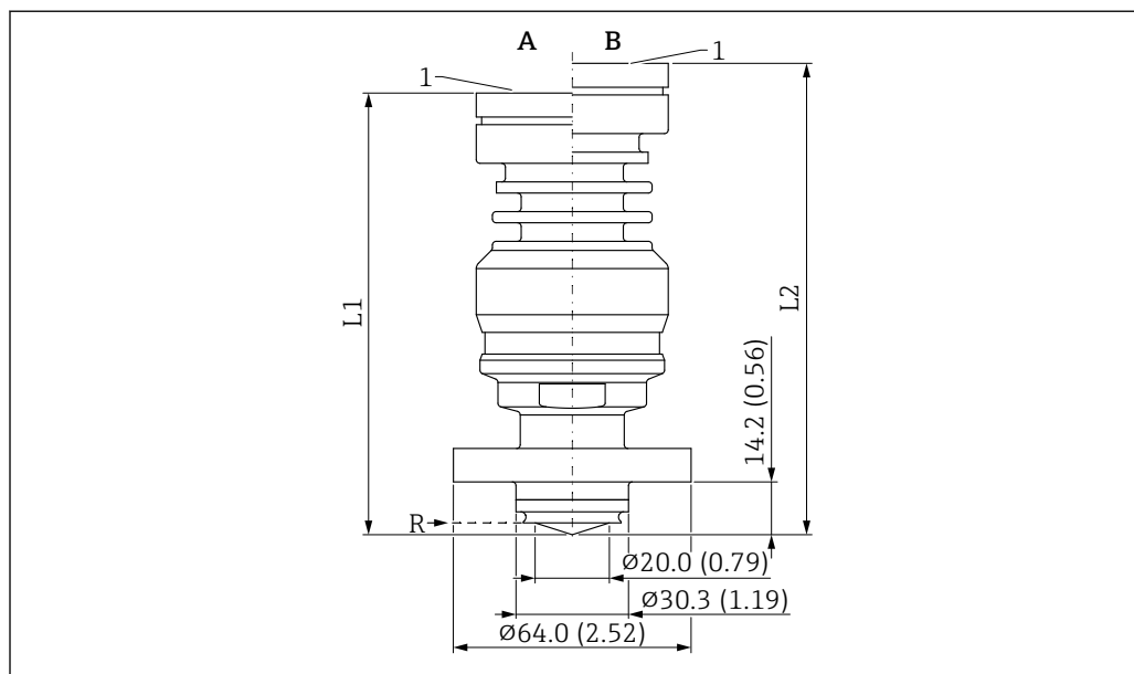
53 Размеры антенны с покрытием, монтаж заподлицо, ПЭЭК, 20 мм (0,75 дюйм), NEUMO BioControl D25. Единица измерения мм (дюйм)
