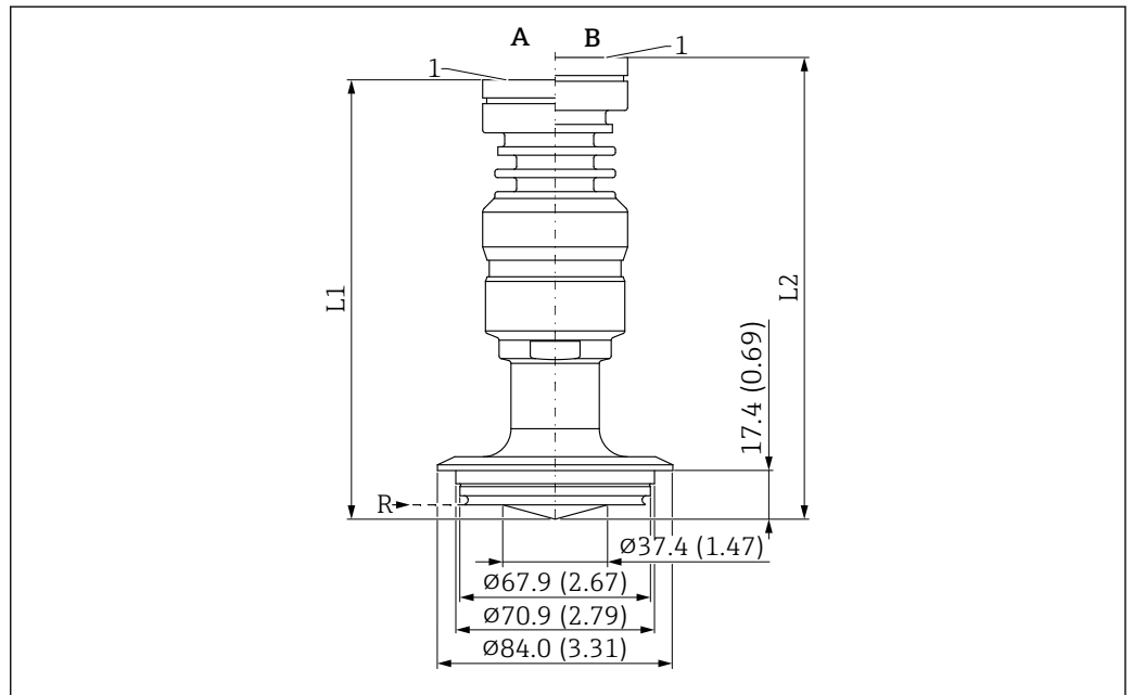
52 Размеры антенны с покрытием, монтаж заподлицо, ПЭЭК, 40 мм (1,5 дюйм), трубка Varivent N, DN65-162. Единица измерения мм (дюйм)
