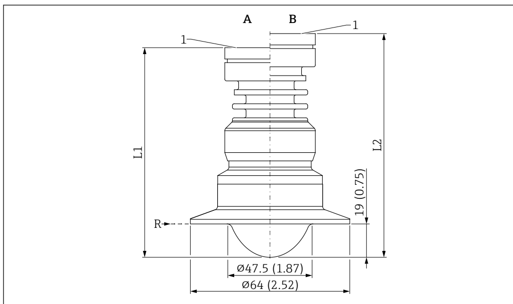
49 Размеры антенны с покрытием из материала PTFE, монтируемой заподлицо, 50 мм (2 дюйм), с соединением Tri-Clamp DN51 (2 дюйма) ISO 2852. Единица измерения мм (дюйм)
