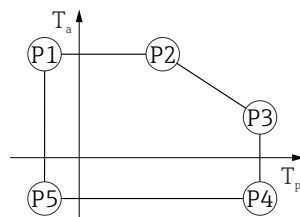
■ 23 Алюминиевый корпус с покрытием; рабочая температура -10 до +200 °C (+14 до +392 °F)
