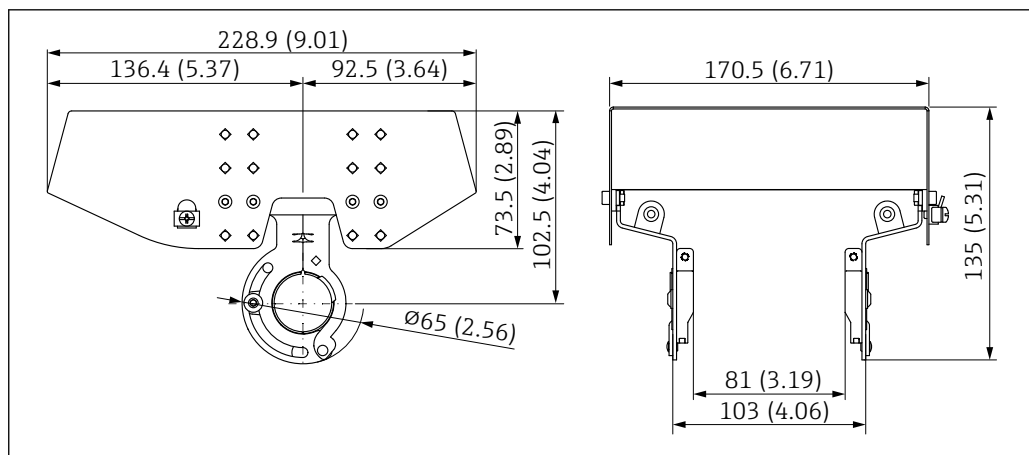
65 Размеры защитного козырька от погодных явлений, сталь 316 L, XW112. Единица измерения мм (дюйм)
