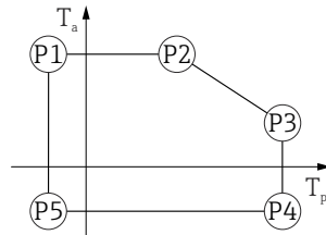
■ 22 Алюминиевый корпус с покрытием; рабочая температура -10 до +150 °C (+14 до +302 °F)
