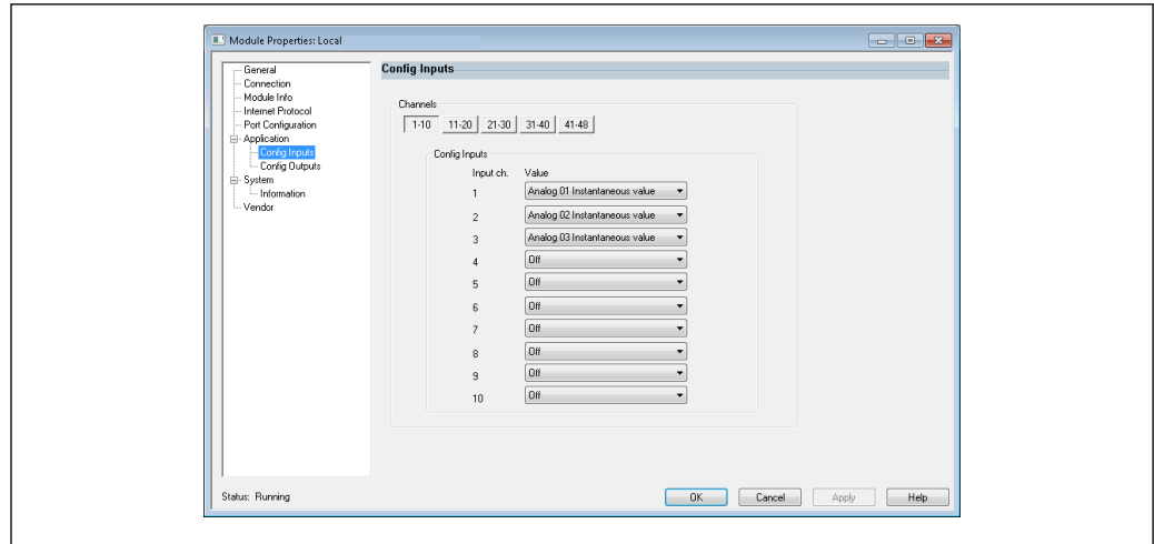
40 Страница Config Inputs
