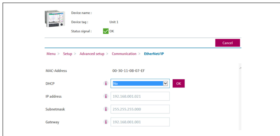
8 Настройки сети: подтверждение изменения (веб-сервер)
