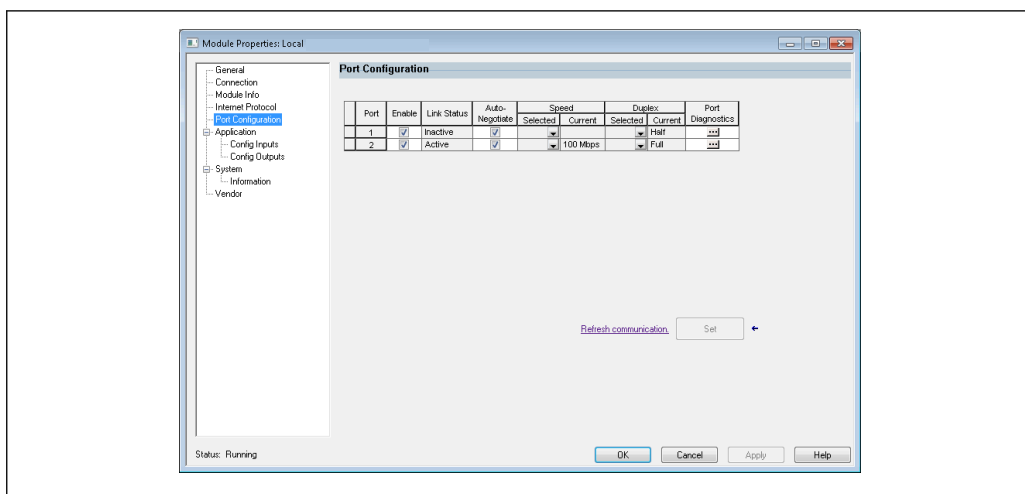
39 Страница конфигурации порта: настройка модуля с несколькими портами
