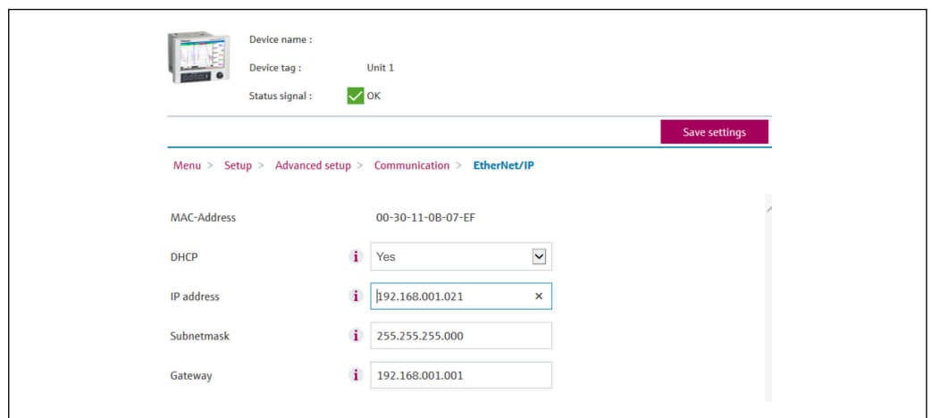
7 Настройки сети: DHCP включен (веб-сервер)
