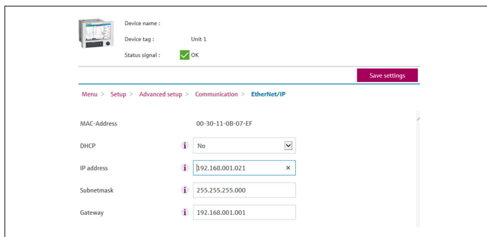
9 Настройки сети: принятие изменения (веб-сервер)
