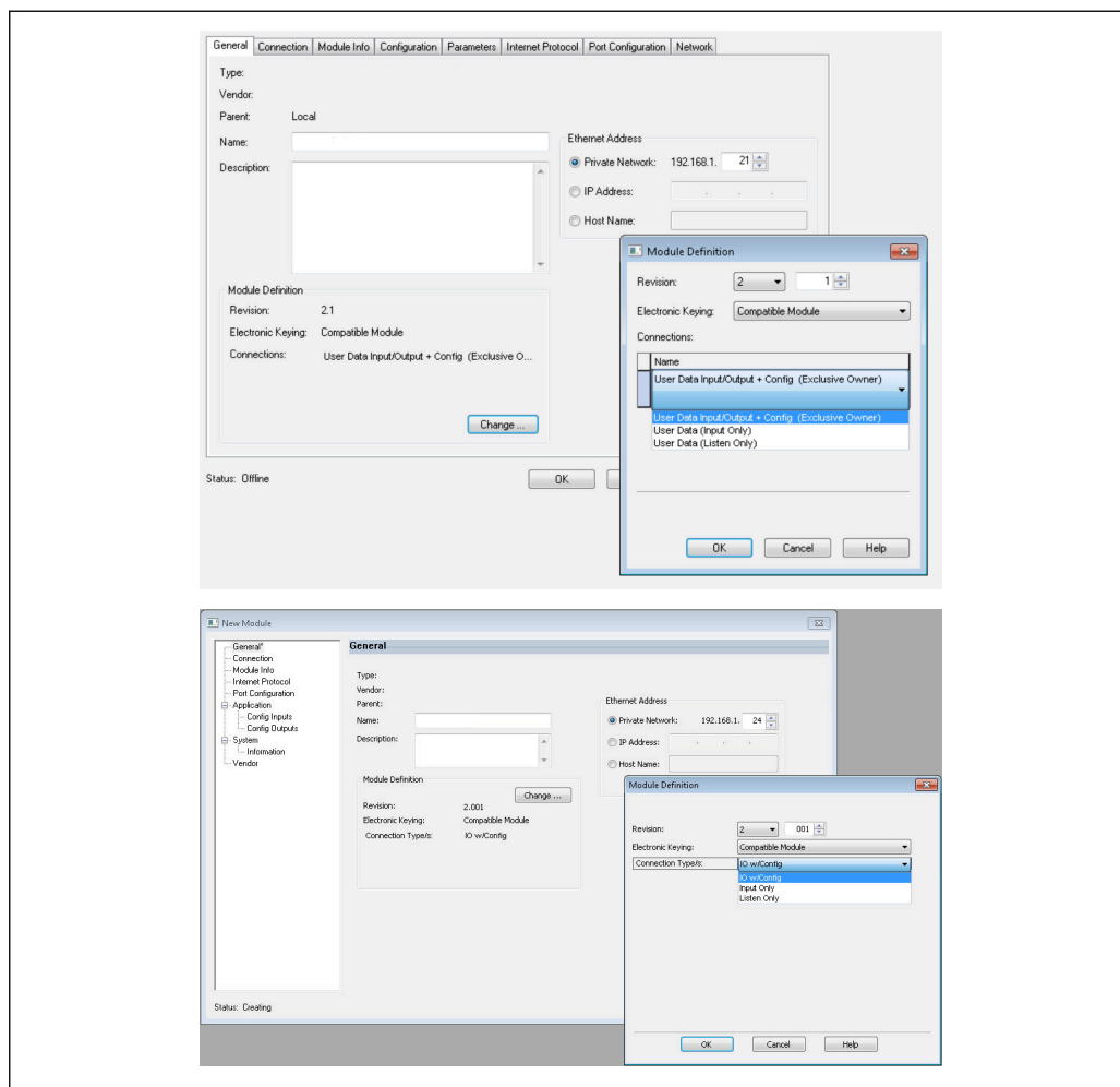
17 Выбор типа подключения (EDS AOP/настраиваемый AOP)
