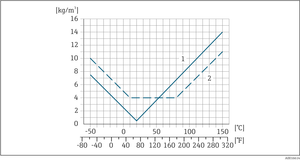
1 Калибровка по плотности на месте эксплуатации, в примере при +20 °C (+68 °F) 2 Специальная калибровка по плотности
