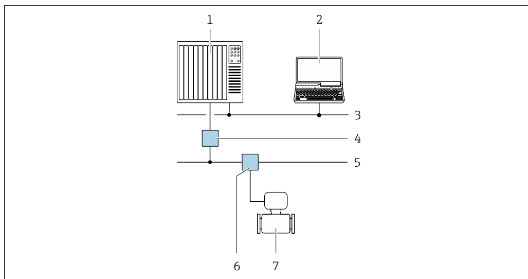
23 Варианты дистанционного управления по сети PROFIBUS PA
