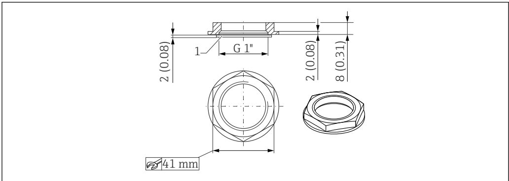
10 Controdamo; dimensioni. Unità di misura mm (in)
