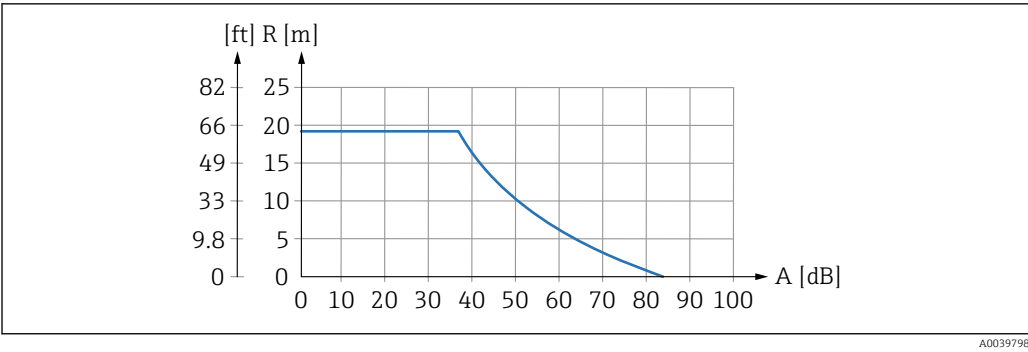
2 Grafico del campo per sensori a ultrasuoni
