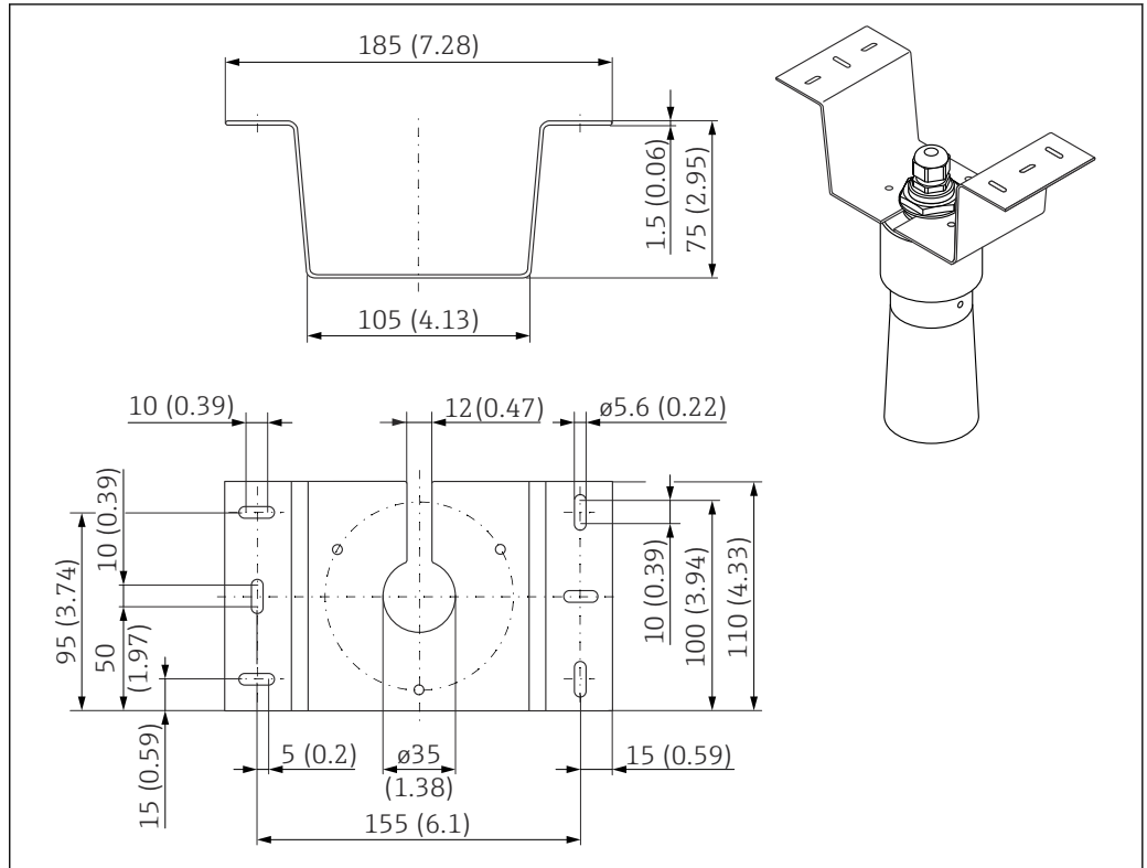
19 Staffa di montaggio per montaggio su soletta. Unità di misura mm (in)
