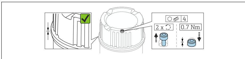
4 Deksel met borgschroef
