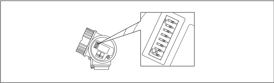
14 Mikroprzełączniki do ustawiania adresu przyrządu w przedziale podłączeniowym
