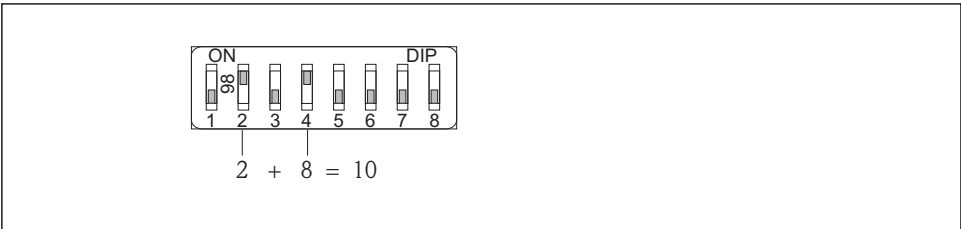
15 Przykład adresacji sprzętowej: mikroprzełącznik 8 w pozycji "OFF"; mikroprzełączniki 1 do 7 służą do ustawienia adresu.
