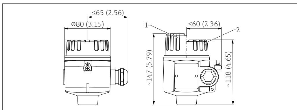
26 Dimensões do invólucro de alumínio, com adaptador aparafusado ao sensor. Unidade de medida mm (in)
