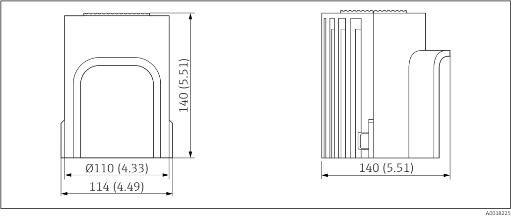
33 Dimensões da tampa de proteção contra intempéries PBT. Unidade de medida mm (in)
