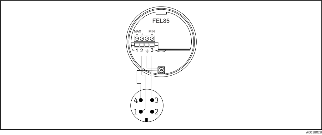
5 Esquema de ligação elétrica com conector M12, modo de detecção de mínimo da operação
