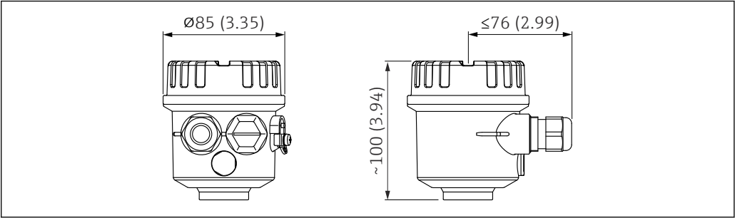
23 Dimensões do invólucro de plástico. Unidade de medida mm (in)
