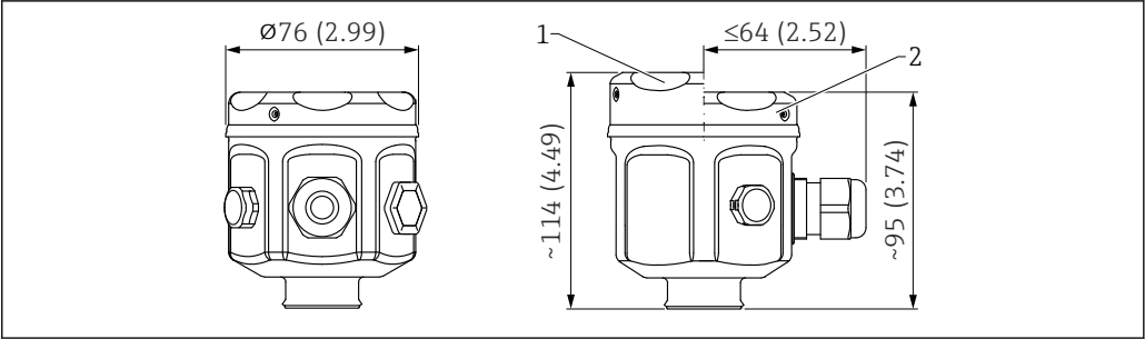
24 Dimensões do invólucro de 316 L, higiênico. Unidade de medida mm (in)
