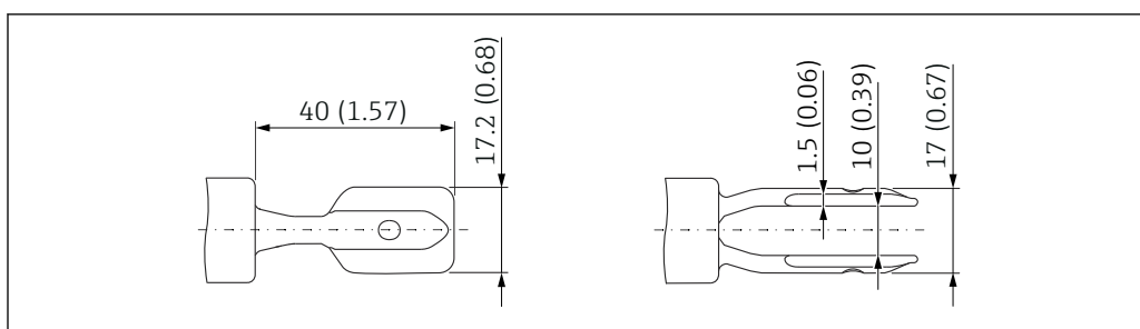
30 Diapasão com revestimento plástico (ECTFE, PFA). Unidade de medida mm (in)
