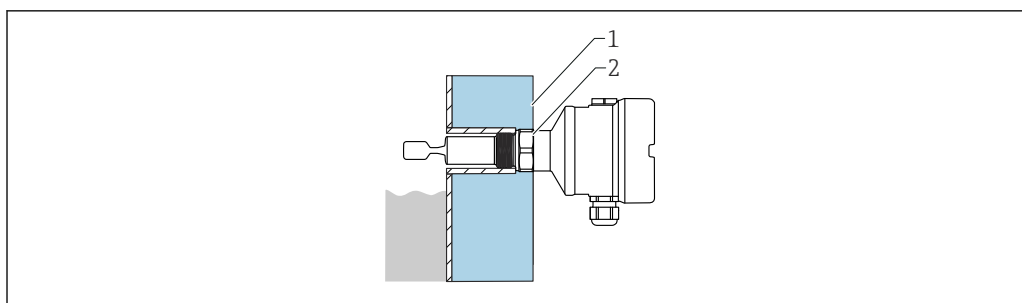
19 Exemplo de um recipiente com isolamento térmico
