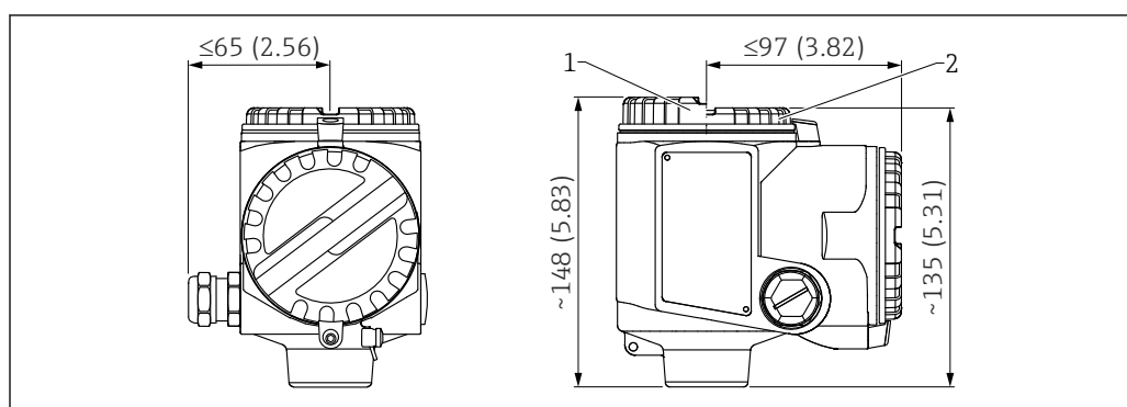
28 Dimensões do invólucro de alumínio com compartimento de terminal separado. Unidade de medida mm (in)
