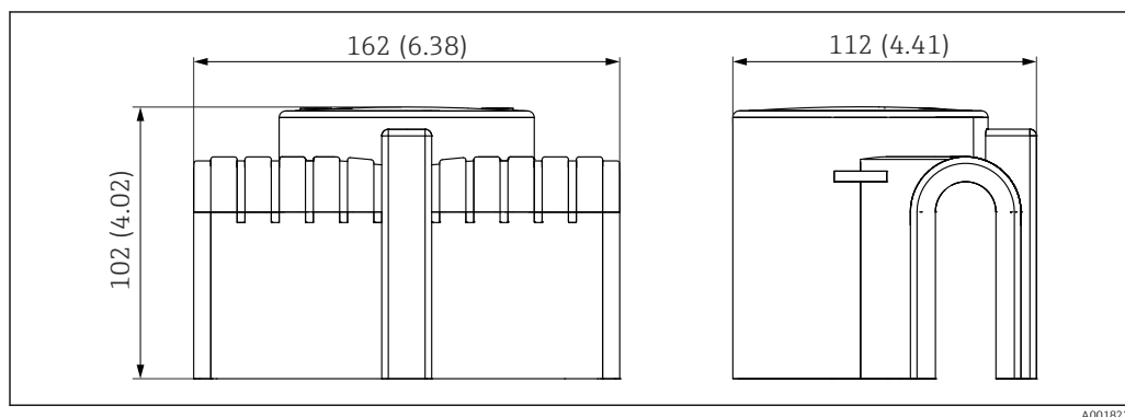
32 Dimensões da tampa de proteção contra intempéries PA6. Unidade de medida mm (in)
