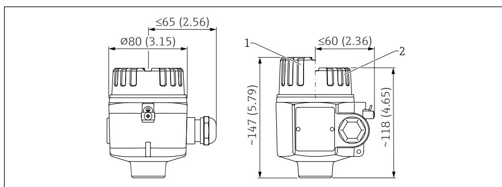
27 Dimensões do invólucro de 316 L, com adaptador aparafusado ao sensor. Unidade de medida mm (in)
