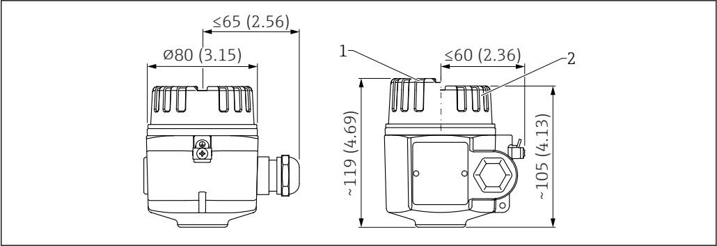
25 Dimensões do invólucro de alumínio. Unidade de medida mm (in)
