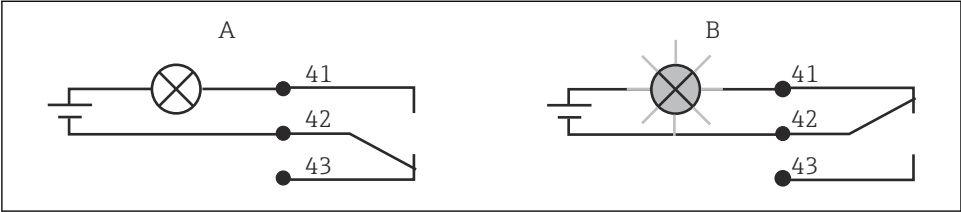
11 Anbefalet fejlsikker afbryder for alarmkontakten
