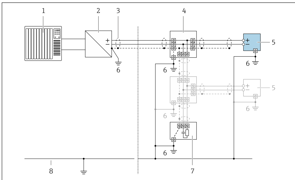
16 Exemple de raccordement pour PROFIBUS PA
