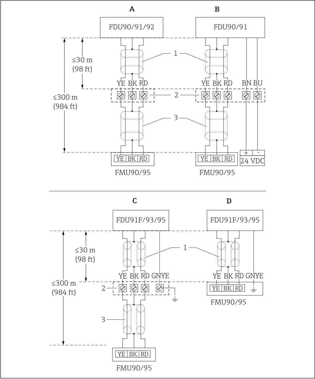
25 Diagramas de conexão para sensores FDU9x; YE: amarelo, BK: preto; RD: vermelho; BU: azul; BN: marrom; GNYE: verde/amarelo
