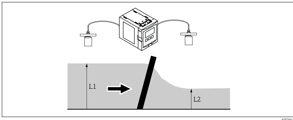
65 Princípio de operação da função de controle rake
