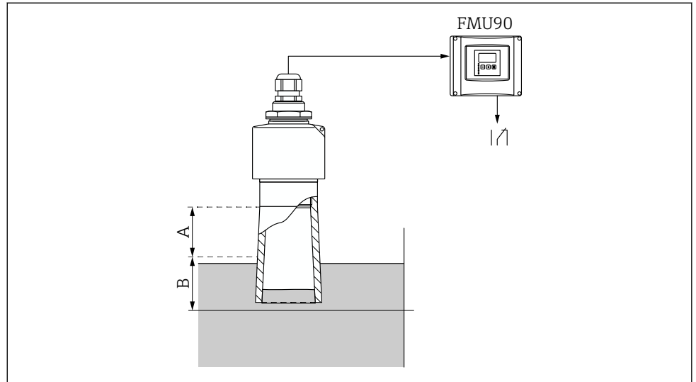
50 Uso do tubo de proteção contra transbordamento para FDU90
