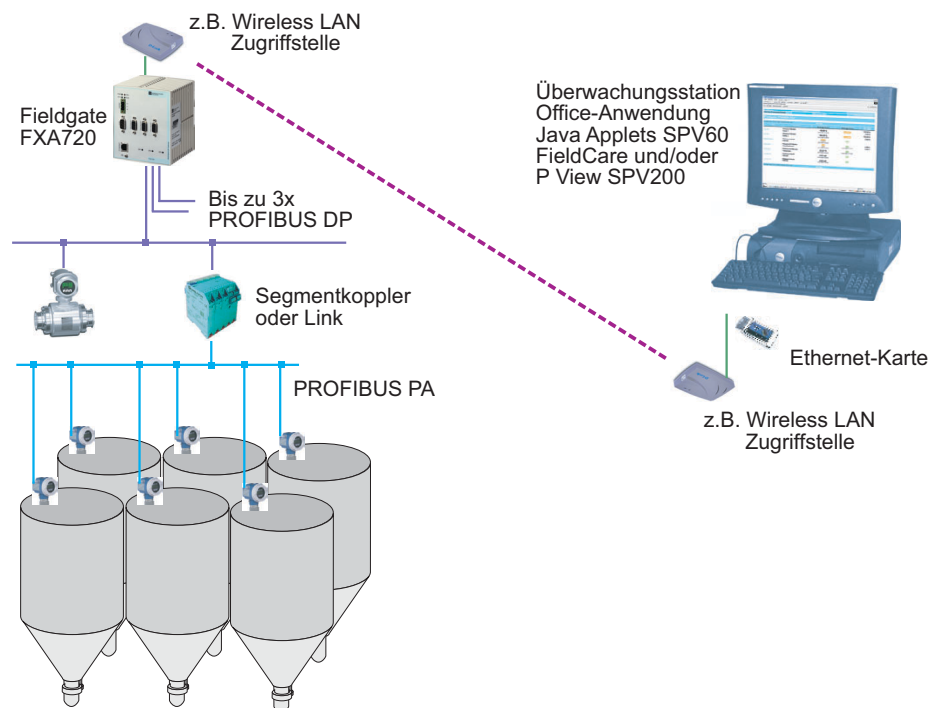
Abb. 3-2: Gewöhnlicher Systemaufbau für Web-basierte Bedien- und Fernüberwachungs-Anwendungen
