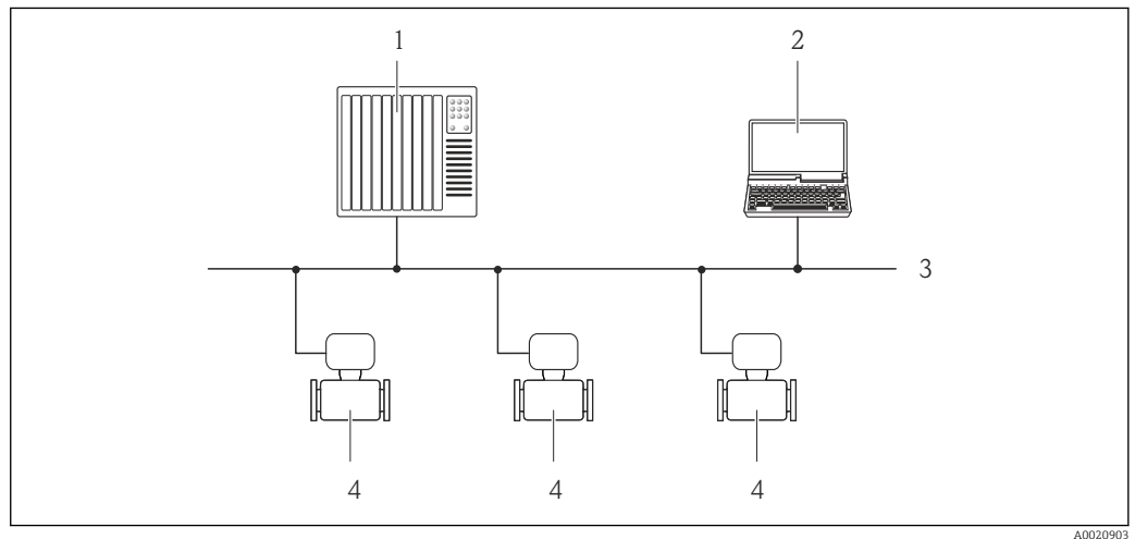
14 Opzioni per il funzionamento a distanza mediante rete PROFIBUS DP
