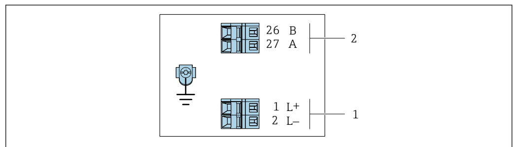
7 Assegnazione dei morsetti PROFIBUS DP
