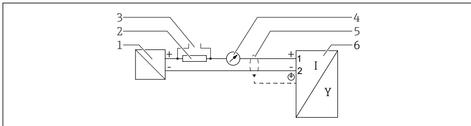
図 3 ブロック図、2線式：4~20 mA HART
