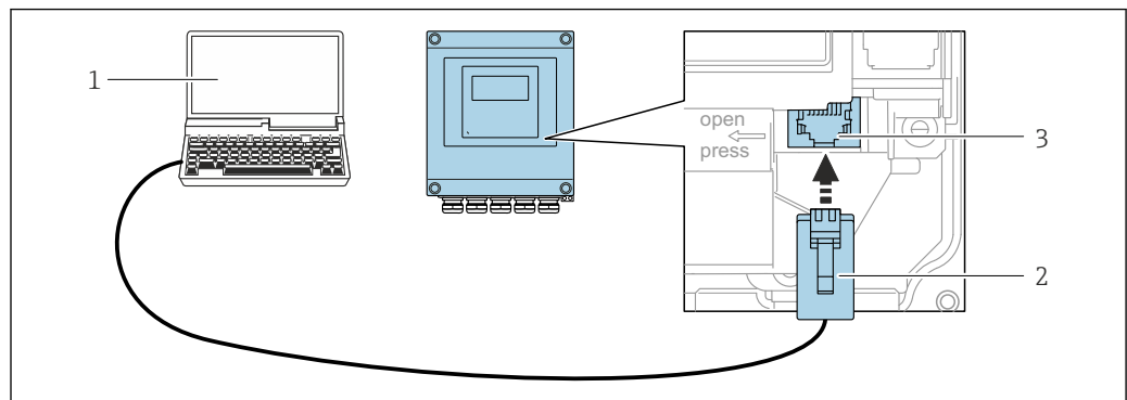
55 Conexión mediante la interfaz de servicio (CDI-RJ45)
