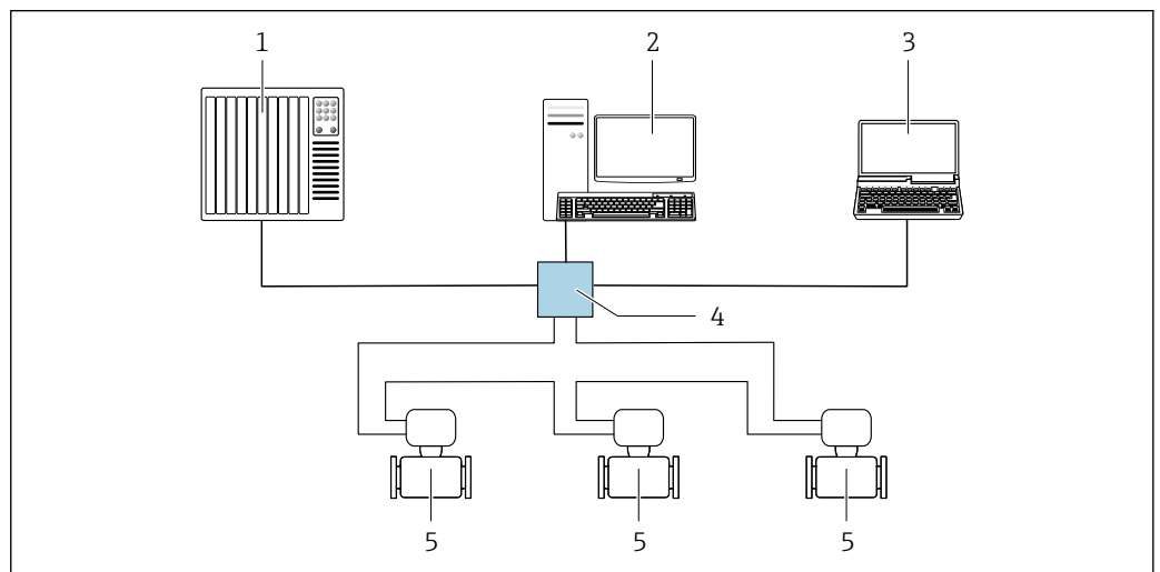
50 Opciones para la configuración a distancia mediante red EtherNet/IP: topología en anillo
