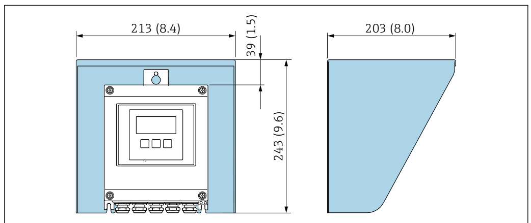
27 Tapa de protección ambiental para Proline 500, digital; unidad mm (in)
