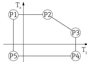
Fig. 18 Invólucro 316L; higiene, temperatura do processo -40 para +130 °C (-40 para +266 °F)
