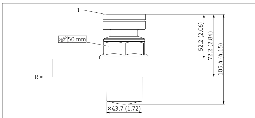
26 Dimensões da antena encapsulada, PVDF, 40 mm (1.5 in), conexão de processo flange UNI. Unidade de medida mm (in)
