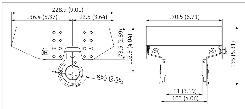
39 Dimensões da tampa de proteção contra tempo, 316 L, XW112. Unidade de medida mm (in)
