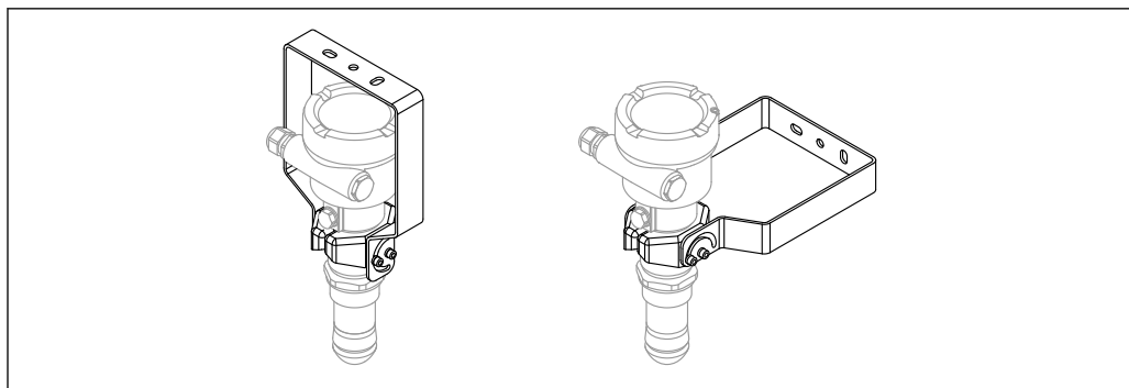
41 Suporte de montagem ajustável FMR6xB; montagem no teto ou em parede
