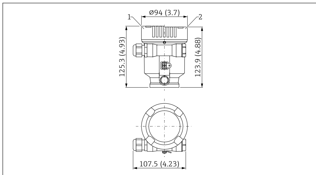
19 Dimensões; invólucro de compartimento único, plástico; incl. acoplamento e conector M20, plástico. Unidade de medida mm (in)
