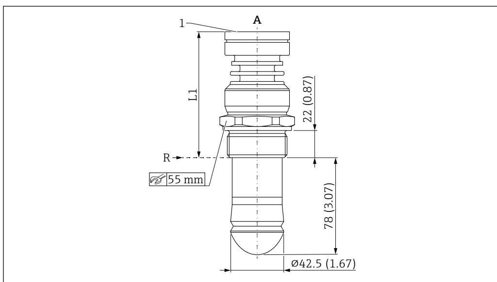
30 Dimensões da antena tipo drip-off 50 mm (2 in), conexão de processo de rosca
