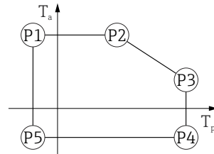
Fig. 17 Invólucro 316L; higiene, temperatura do processo -40 para +80 °C (-40 para +176 °F)
