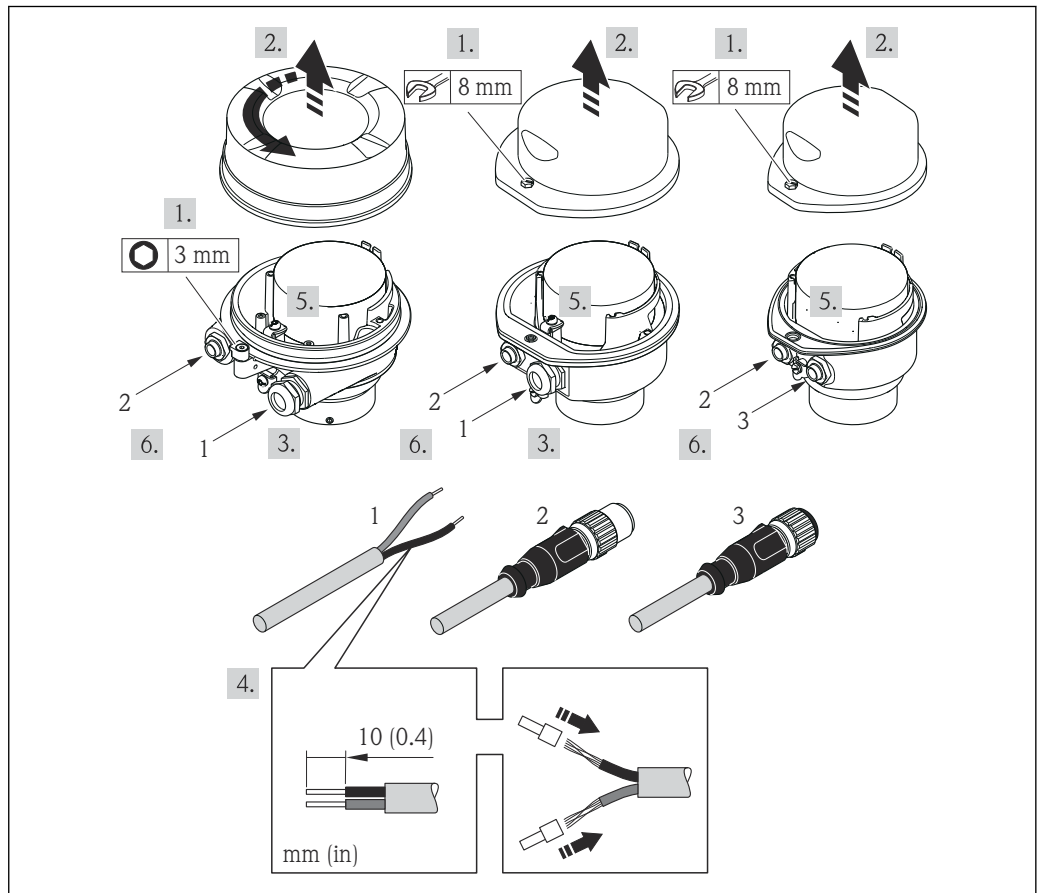
图 10 设备类型和连接实例
