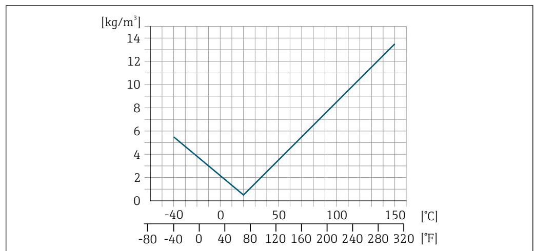
16 现场密度校正，例如在 +20 \text{ }^\circ\text{C} ( +68 \text{ }^\circ\text{F} ) 时
