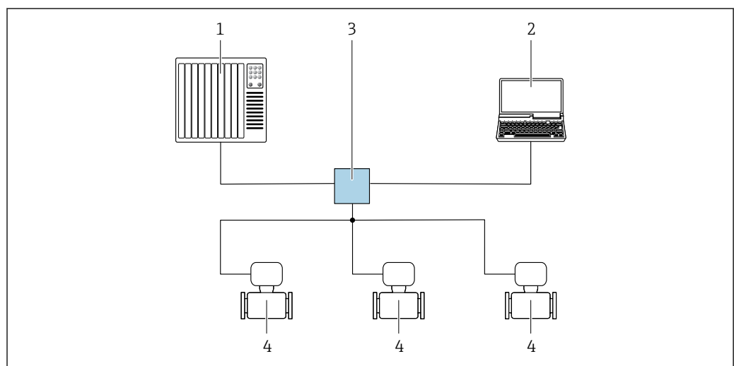
图 19 通过 PROFINET 网络进行远程操作：星形拓扑结构
