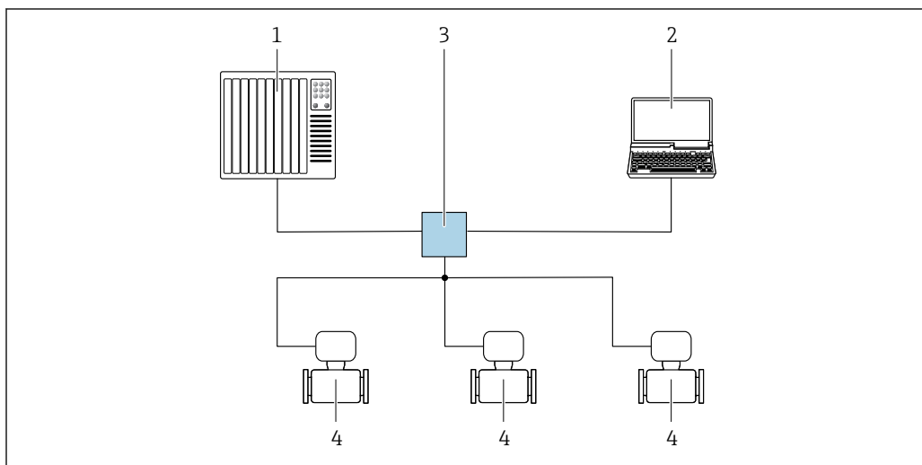
图 13 通过 PROFINET 网络进行远程操作：星形拓扑结构
