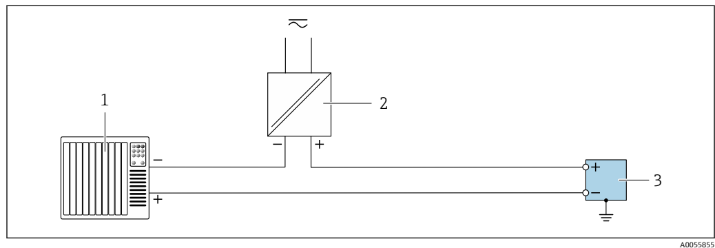
图 11 接线实例：脉冲输出/频率输出/开关量输出（无源）
