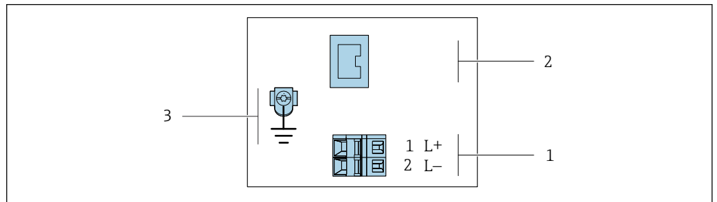
图 8 PROFINET 型仪表的接线端子分配
