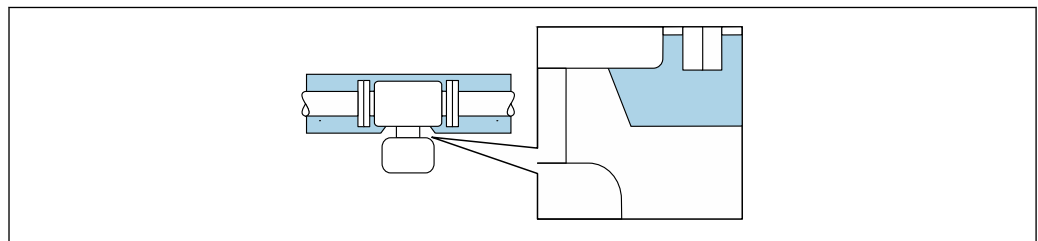
19 Isolation thermique avec tube prolongateur exposé
