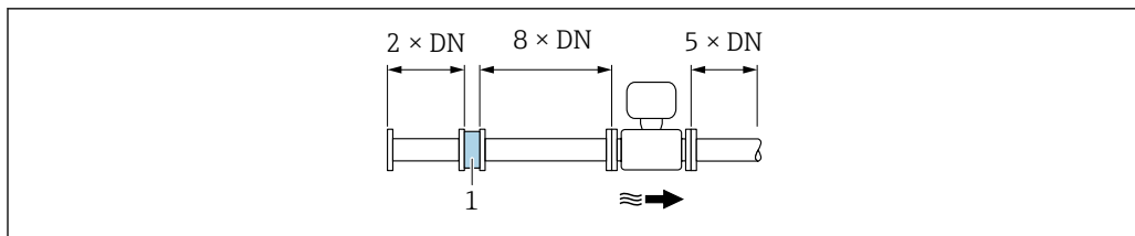
1 Strömungsgleichrichter
