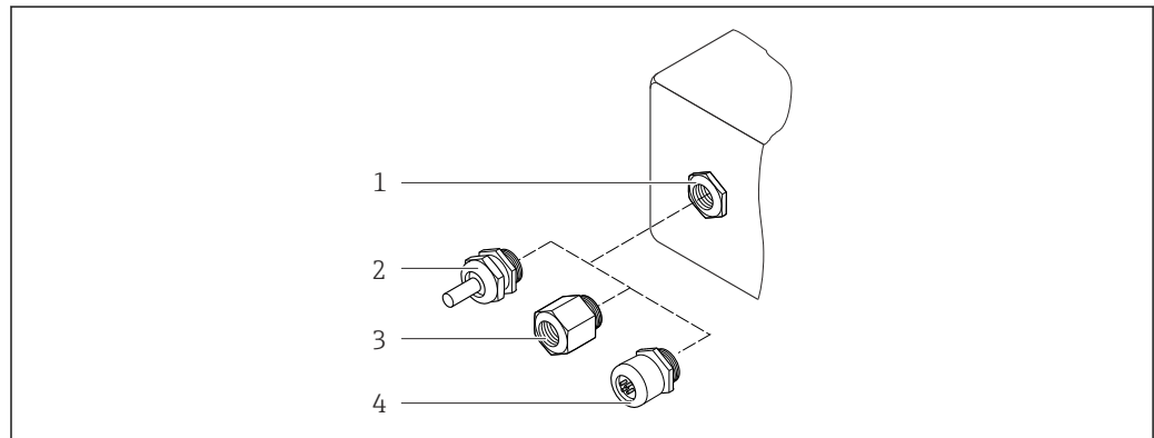
27 Mögliche Kabeleinführungen/-verschraubungen
