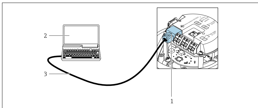
37 Подключение для кода заказа «Выход», опция B «4-20 мА HART, импульсный/частотный/релейный выход»
