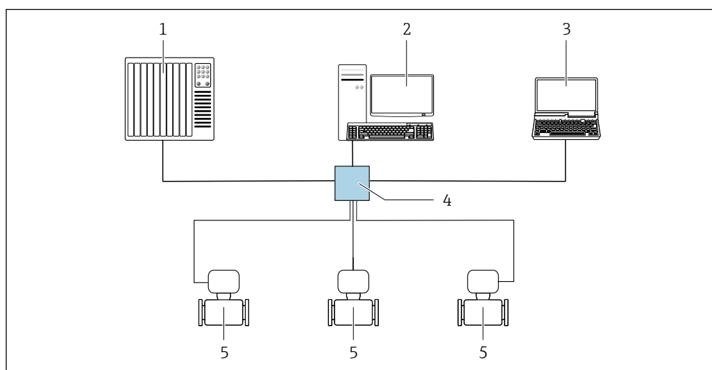
▣ 35 Варианты дистанционного управления через сеть EtherNet/IP: топология «звезда»
