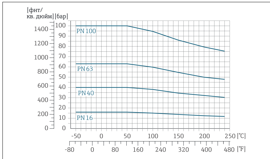
16 С материалом фланца 1.4404 (F316/F316L), сплав Alloy C22
