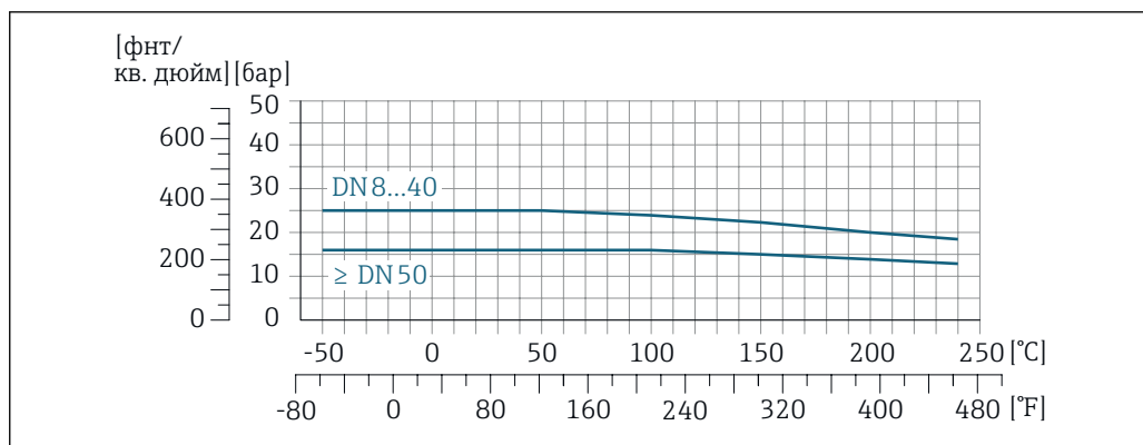
20 С материалом присоединения 1.4404 (316/316L)
