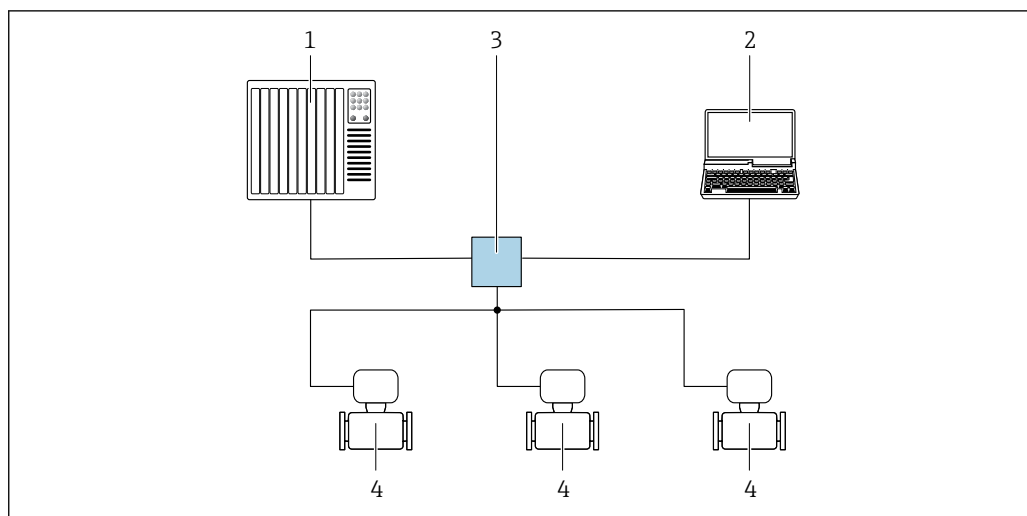
36 Варианты дистанционного управления через сеть PROFINET: топология «звезда»
