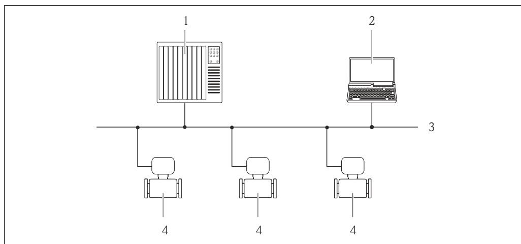
▣ 34 Варианты дистанционного управления через сеть PROFIBUS DP
