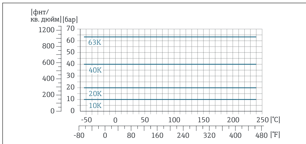
19 С материалом фланца 1.4404 (F316/F316L), сплав Alloy C22
