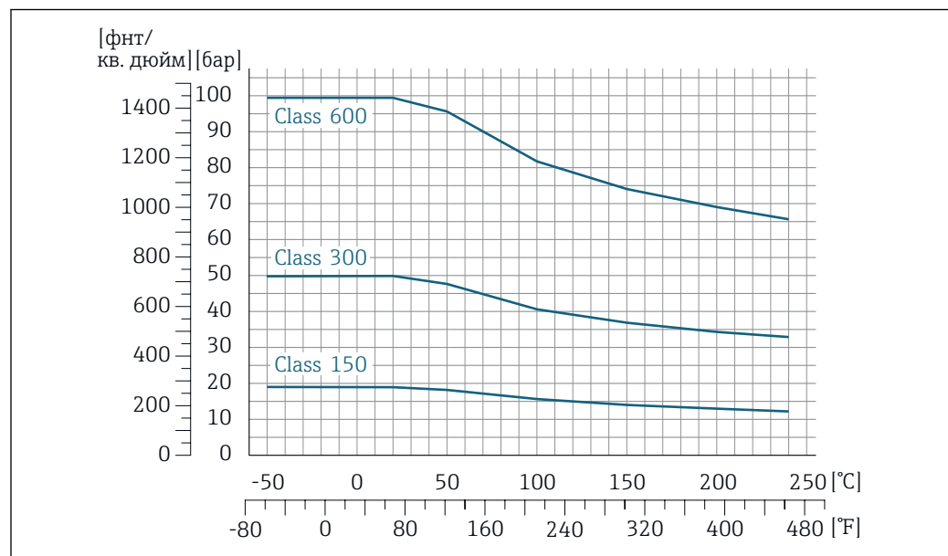
22 С материалом фланца 1.4301 (F304); смачиваемые компоненты: сплав Alloy C22
