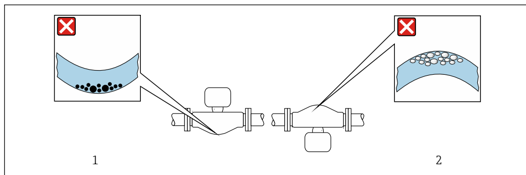
☒ 13 Монтажное положение датчика с изогнутой измерительной трубкой
