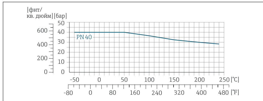
21 С материалом фланца 1.4301 (F304); смачиваемые компоненты: сплав Alloy C22
