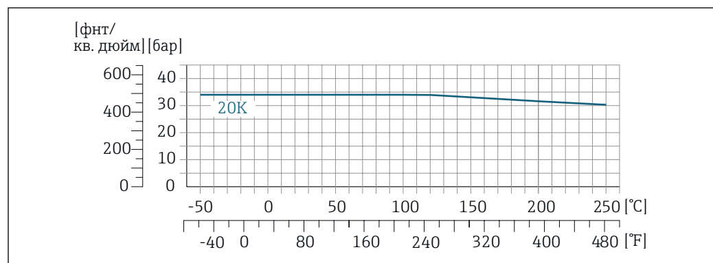
23 С материалом фланца 1.4301 (F304); смачиваемые компоненты: сплав Alloy C22
