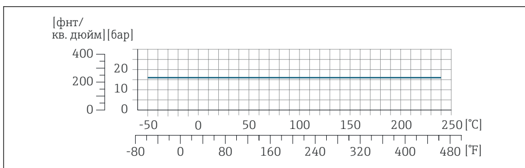
27 С материалом присоединения 1.4404 (316/316L)
