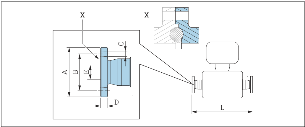
Bride fixe DIN 11864-2
