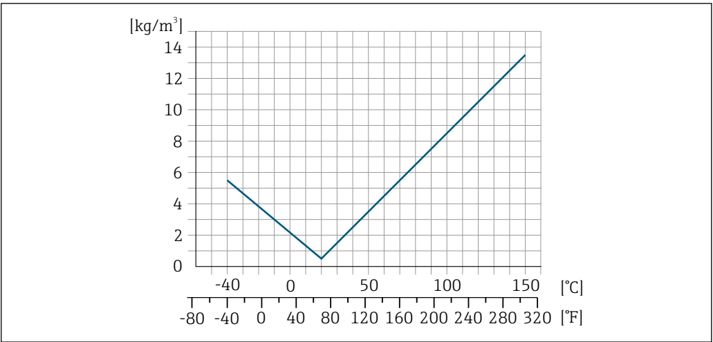
13 Ajustage sur site de la masse volumique, par exemple à +20^\circ\text{C} ( +68^\circ\text{F} )
