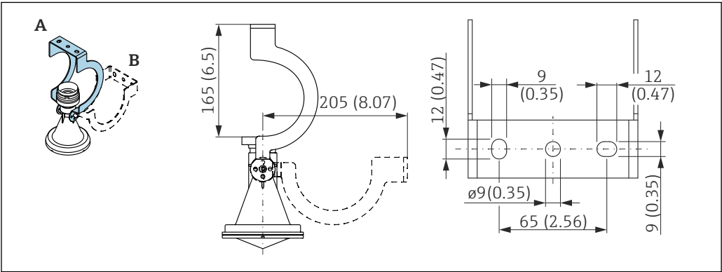
図 30 取付ブラケットの寸法。測定単位 mm (in)
