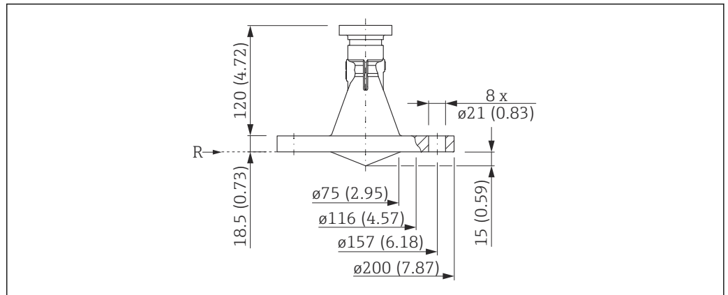
31 スリップオンフランジ 3"/DN80 付き FMR56 の寸法。測定単位 mm (in)
