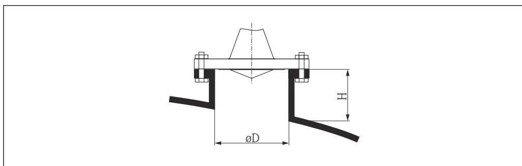
図 20 スリップオンフランジ付きホーンアンテナのノズル径とノズル高
