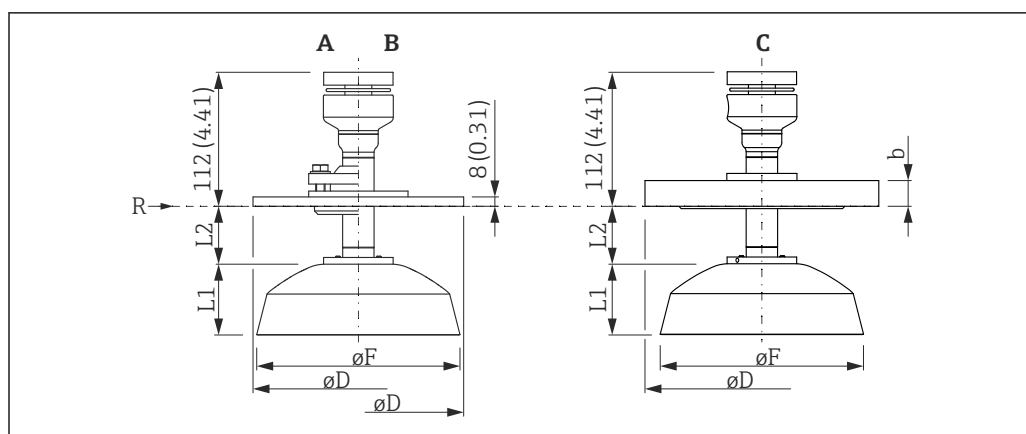
図 36 パラボラアンテナ付き FMR57 の寸法 (単位: mm (in))
