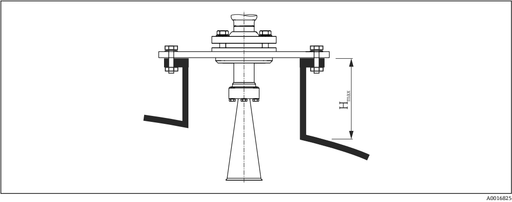
22 ホーンアンテナのノズル高 (FMR57)
