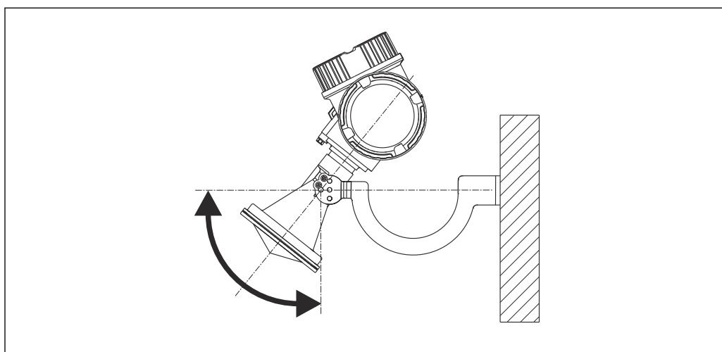
図 21 取付ブラケット付きホーンアンテナの取付け
