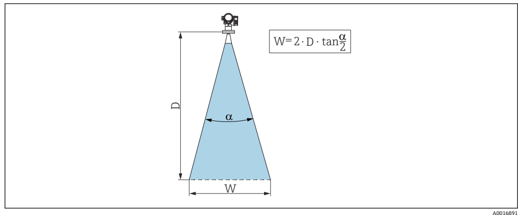
図 19 放射角 \alpha 、距離 D 、ビーム幅 W の関係
