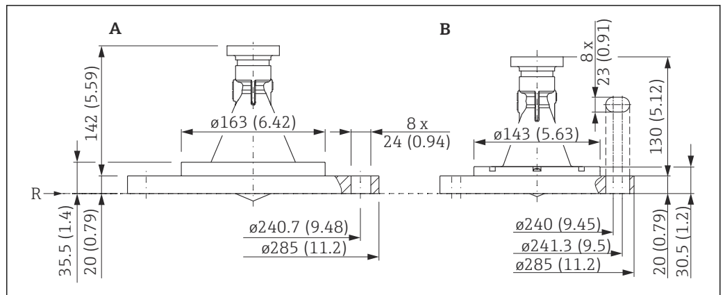
図 33 スリップオンフランジ 6"/DN150 付き FMR56 の寸法。測定単位 mm (in)
