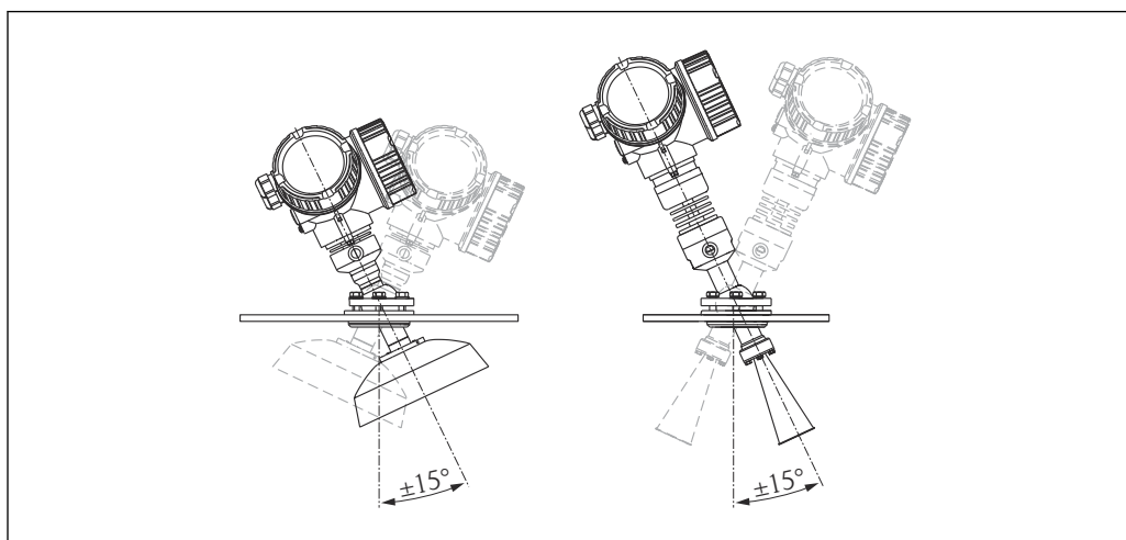
図 24 角度調節器付き Micropilot FMR57
