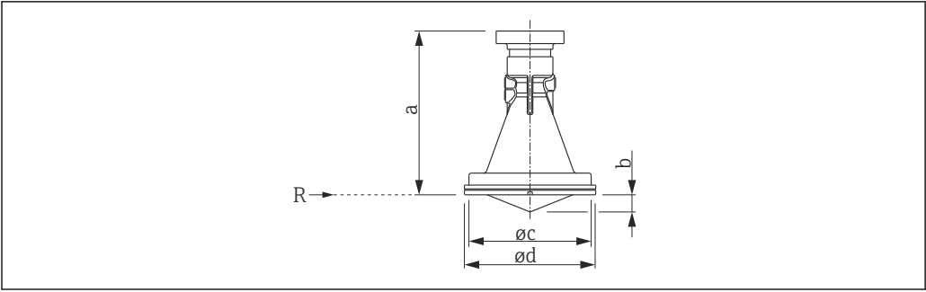
図 29 FMR56 の寸法（プロセス接続部なし）。測定単位 mm (in)
