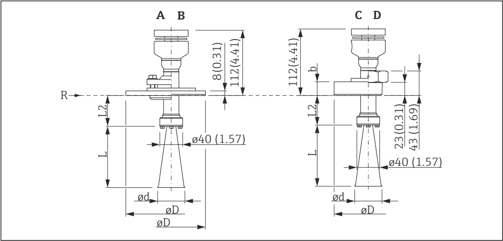
図 34 ホーンアンテナ（標準バージョン）付き FMR57 の寸法。測定単位 mm (in)
