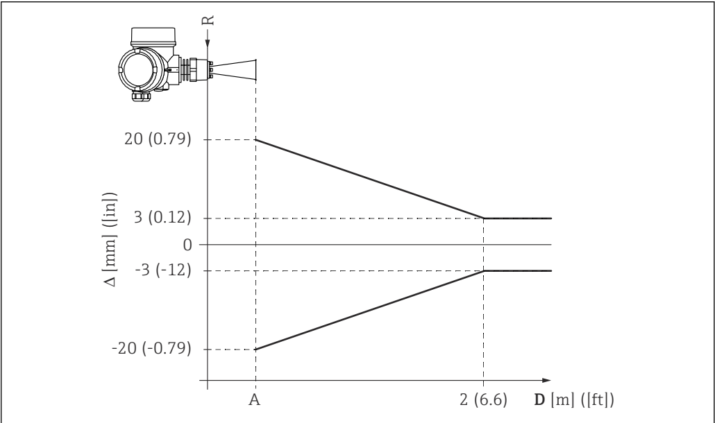
図 18 近範囲アプリケーションにおける最大測定誤差
