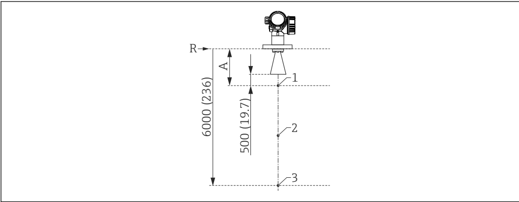
図 46 3 点リニアリティプロトコルの各点、使用単位：mm (in)
