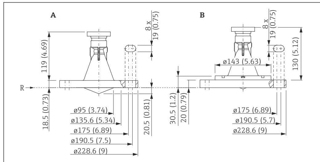
図 32 スリップオンフランジ 4"/DN100 付き FMR56 の寸法。測定単位 mm (in)
