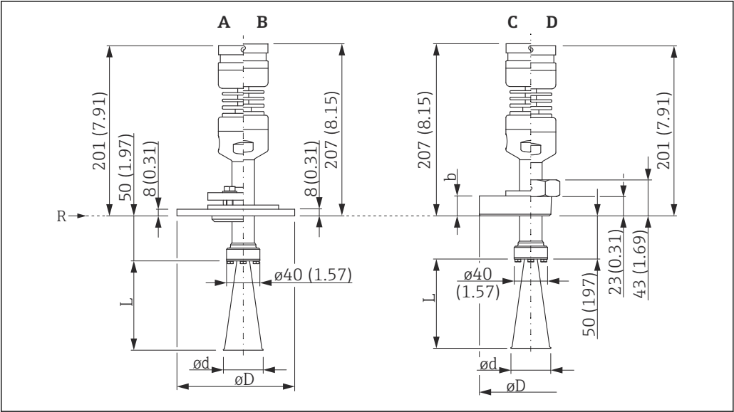
35 ホーンアンテナ（高温バージョン）付き FMR57 の寸法（単位：mm (in)）
