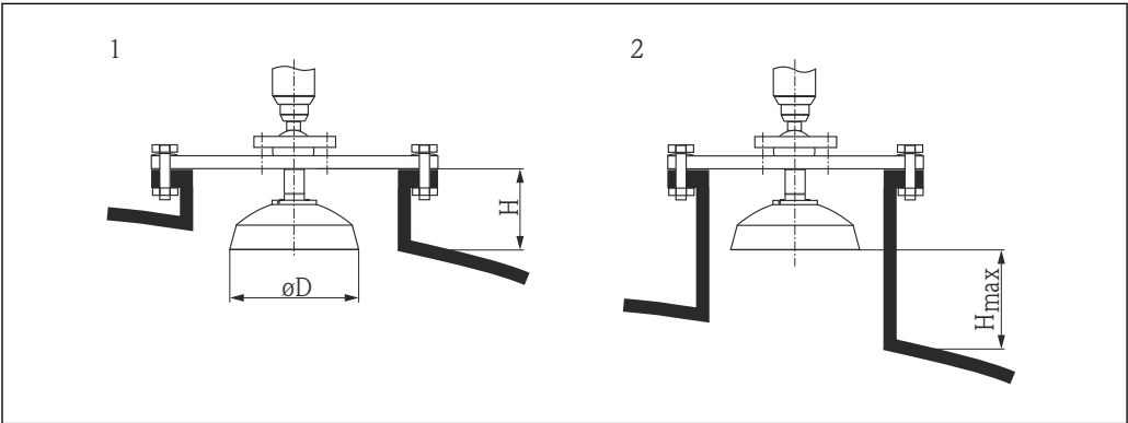
図 23 パラボラアンテナ付き Micropilot FMR57 のノズル取付け
