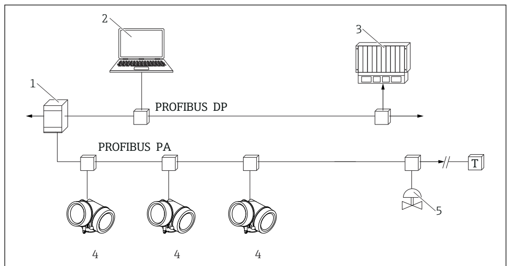
図 41 PROFIBUS PA プロトコルを介したリモート操作用のオプション
