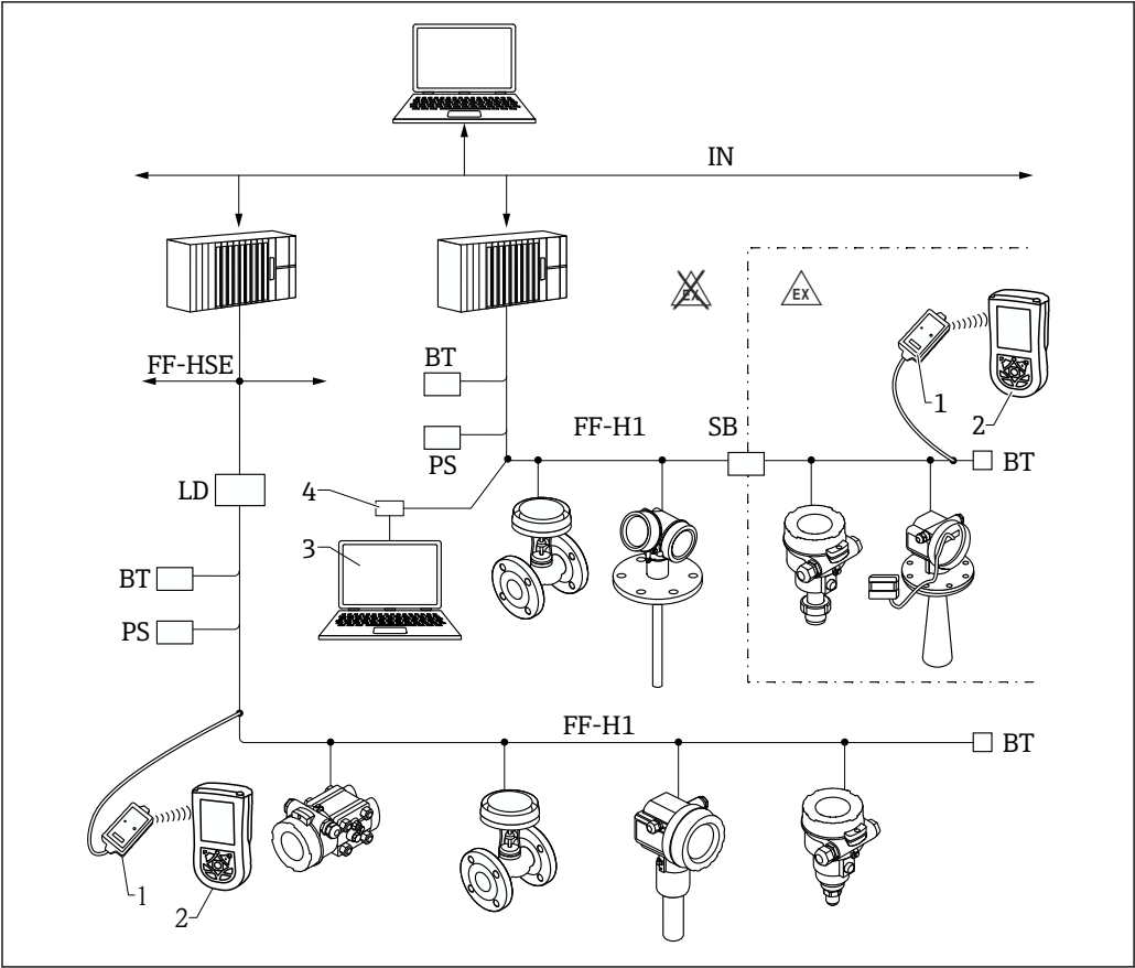
図 42 FOUNDATION フィールドバスシステム構成および関連するコンポーネント
