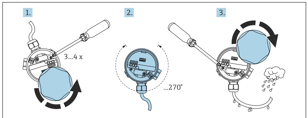
図 17 ハウジング（ロックネジ付き）、ケーブルにドリップループを設けます。
