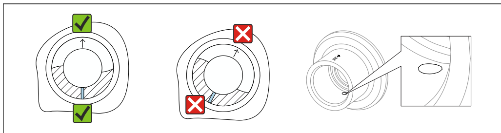
図 21 漏れ検知用の穴付きの溶接アダプタ
