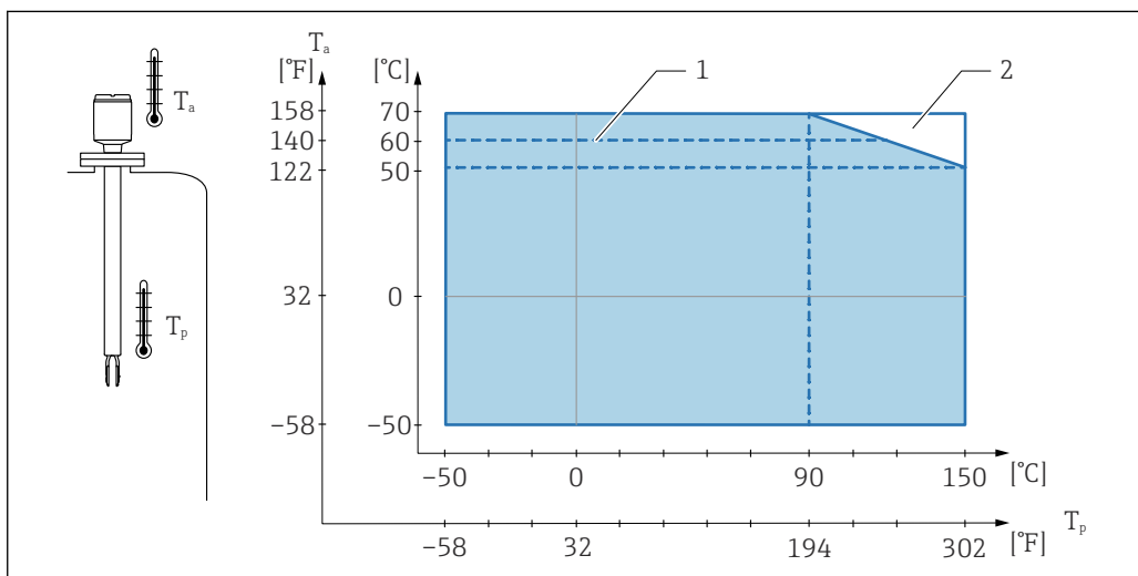
図 22 容器内のプロセス温度 T_p に応じたハウジングの許容周囲温度 T_a 、最高プロセス温度 150 °C (302 °F)
