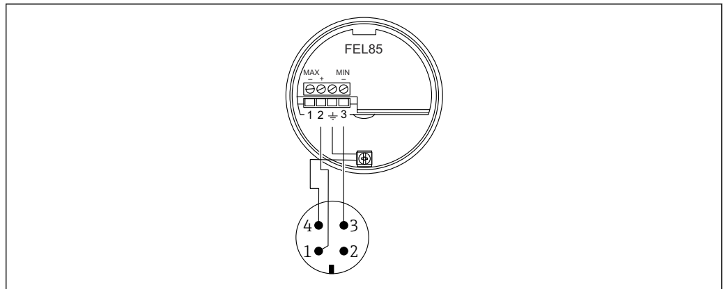
図 5 M12 コネクタを使用した端子の割当て、下限検知動作モード
