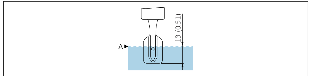
図 8 基準動作条件下のスイッチポイント。測定単位 mm (in)
