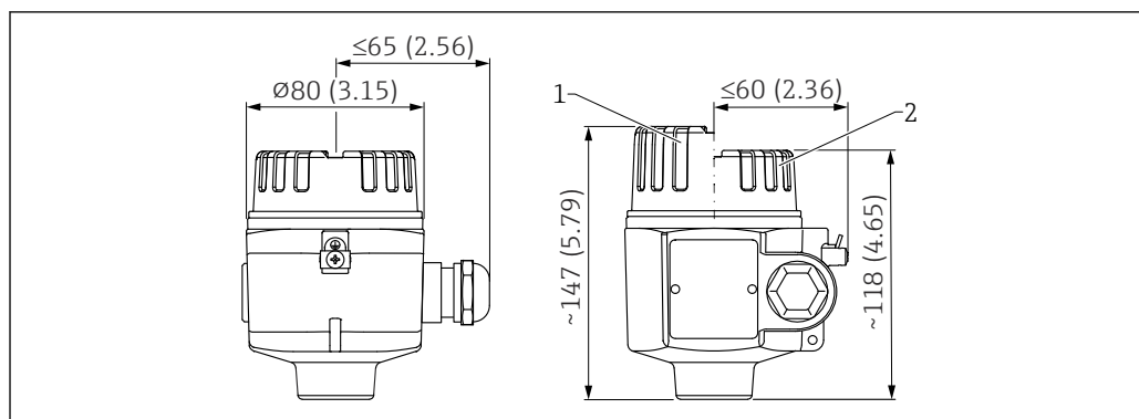
図 30 アルミニウムハウジングの寸法、センサへのネジ込みアダプタ付き。測定単位 mm (in)
