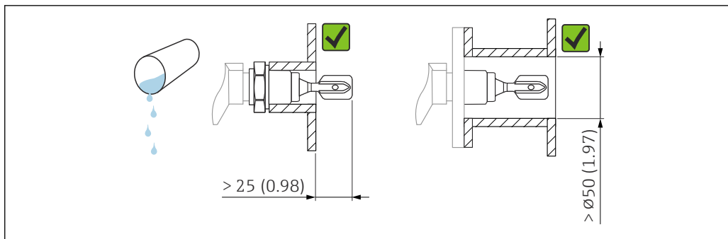
図 11 低粘度液体での設置例。測定単位 mm (in)
