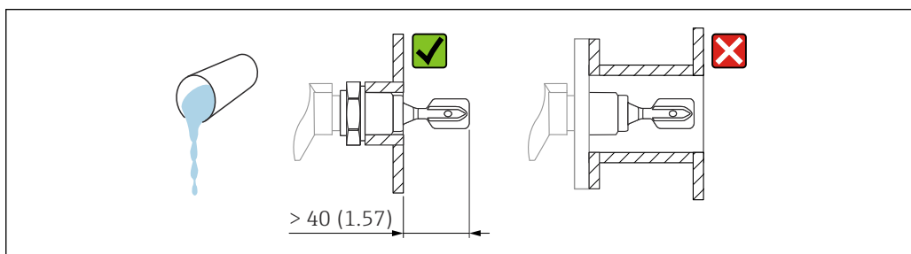
図 12 高粘度液体での設置例。測定単位 mm (in)
