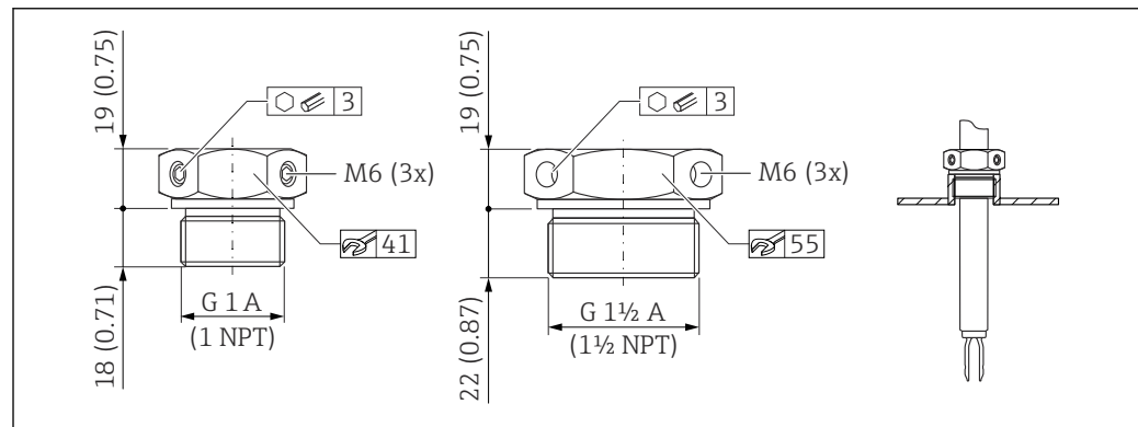
図 40 スライディングスリーブ (大気圧用 : p_e = 0 MPa (0 psi))。測定単位 mm (in)
