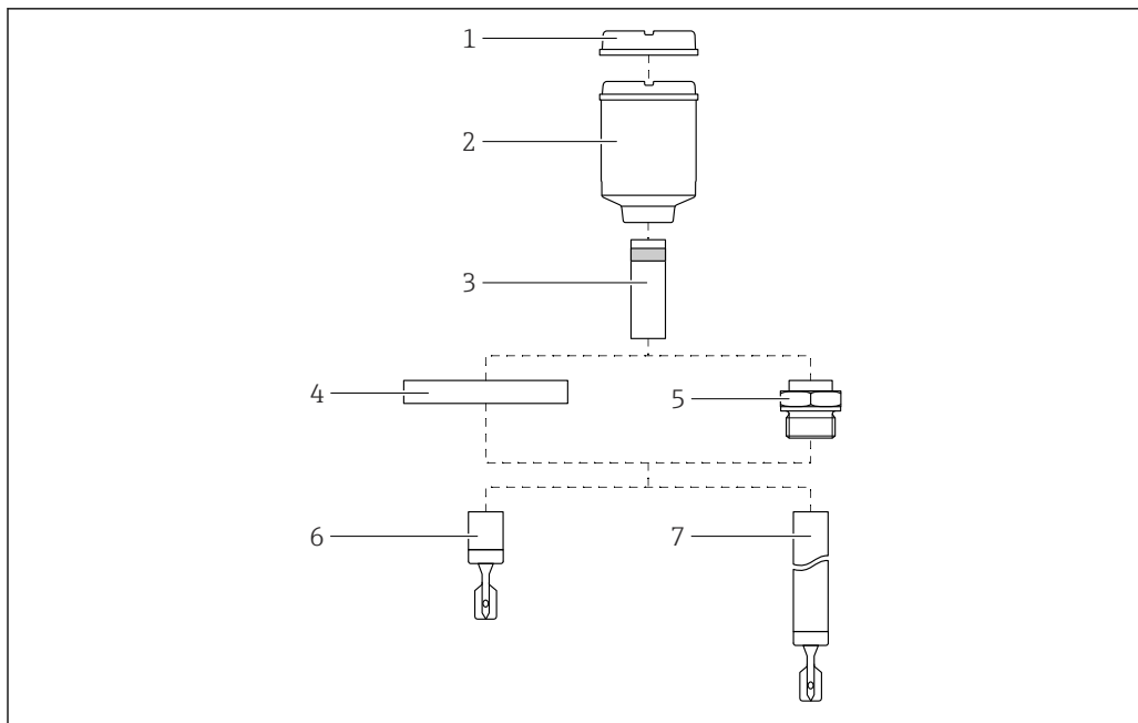
図 26 本体高さを特定するための構成品
