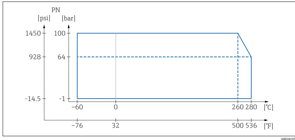
図 25 高温バージョン (230°C (450°F)/280°C (540°F)) のプロセス圧力範囲
