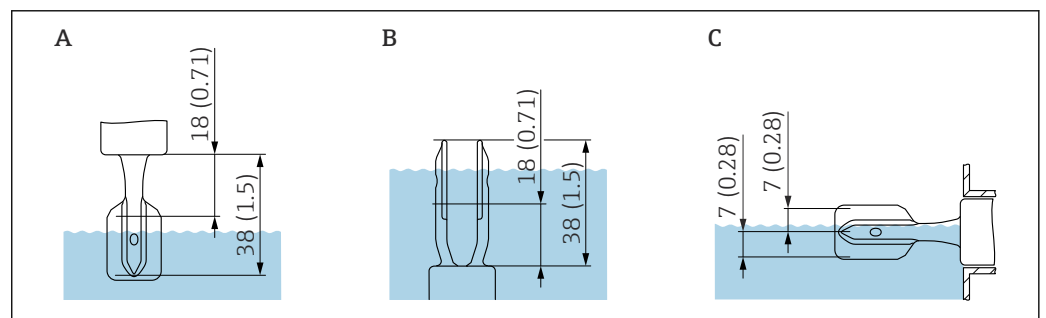
図 9 スイッチポイント（取付方向に応じて異なる）。測定単位 mm (in)
