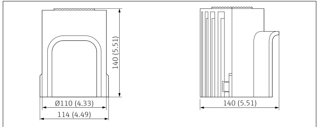
図 38 日除けカバー PBT の寸法。測定単位 mm (in)
