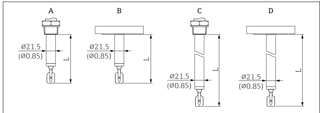
図 33 センサ長 L。測定単位 mm (in)
