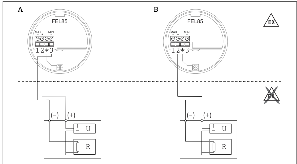
図 7 PLC との接続
