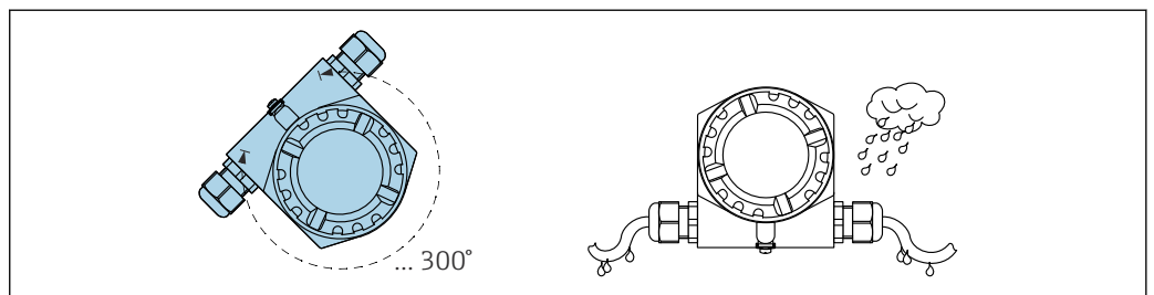
図 18 ハウジング（ロックネジなし）、ケーブルにドリップループを設けます。
