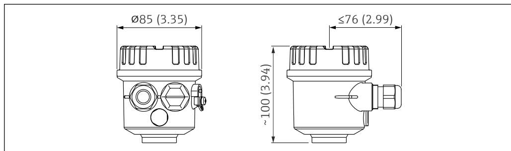
図 27 プラスチックハウジングの寸法。測定単位 mm (in)
