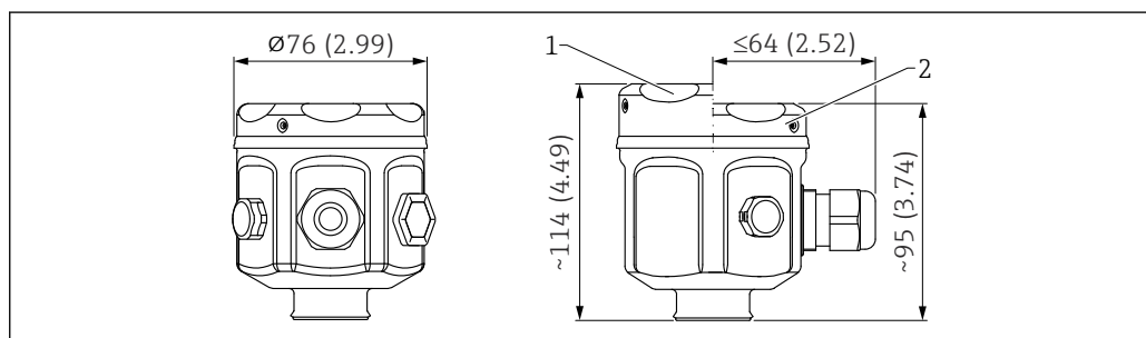
図 28 SUS 316L 相当製ハウジング、サニタリ仕様の寸法。測定単位 mm (in)
