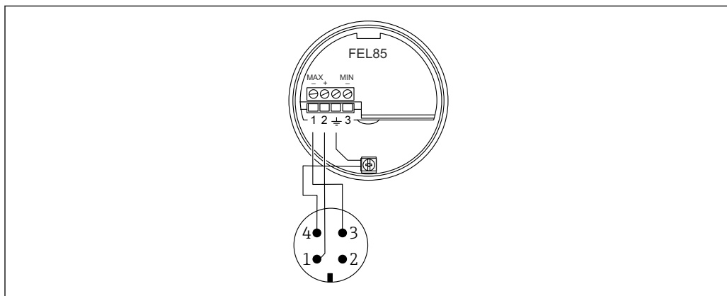
図 4 M12 コネクタを使用した端子の割当て、上限検知動作モード
