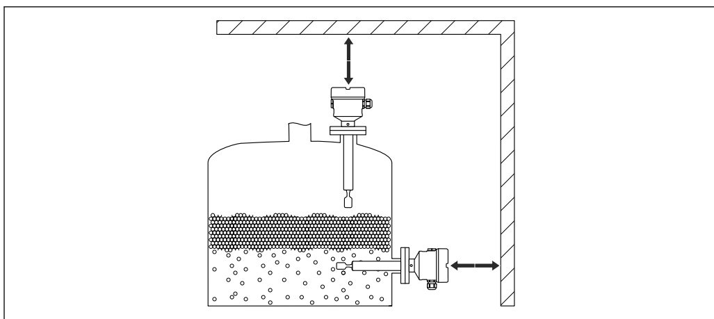
図 14 タンク外部の間隔を考慮すること
