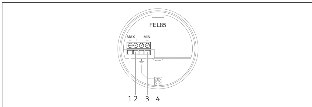
図 2 端子部の接続端子と接地端子
