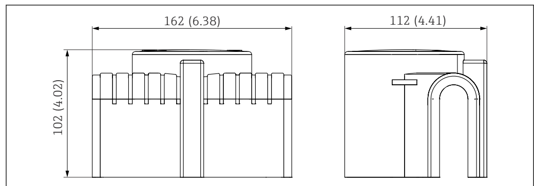
図 37 日除けカバー PA6 の寸法。測定単位 mm (in)
