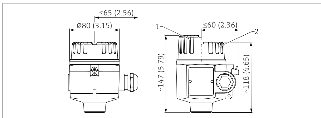
図 31 SUS 316L 相当製ハウジングの寸法、センサへのネジ込みアダプタ付き。測定単位 mm (in)
