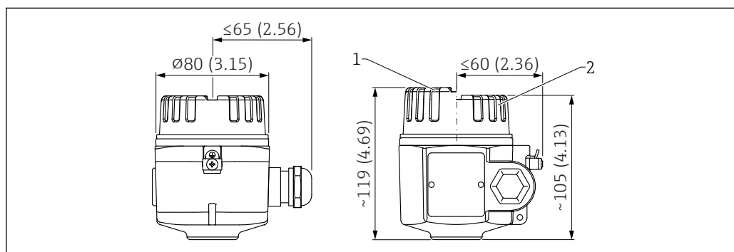
図 29 アルミニウムハウジングの寸法。測定単位 mm (in)
