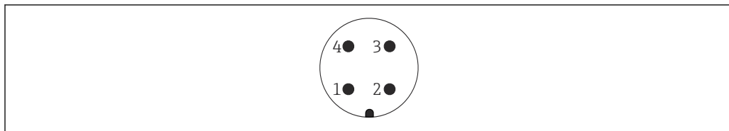
図 3 M12 プラグ、ピンの割当て
