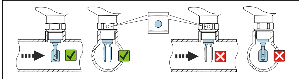
図 16 パイプへの設置（音叉部の位置とマークを考慮します）
