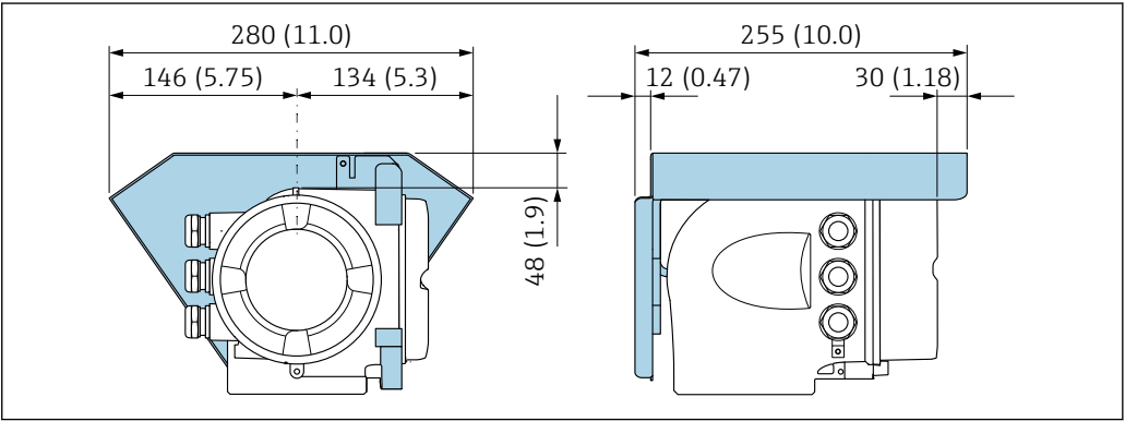
40 Proline 500 用の日除けカバー、単位 mm (in)
