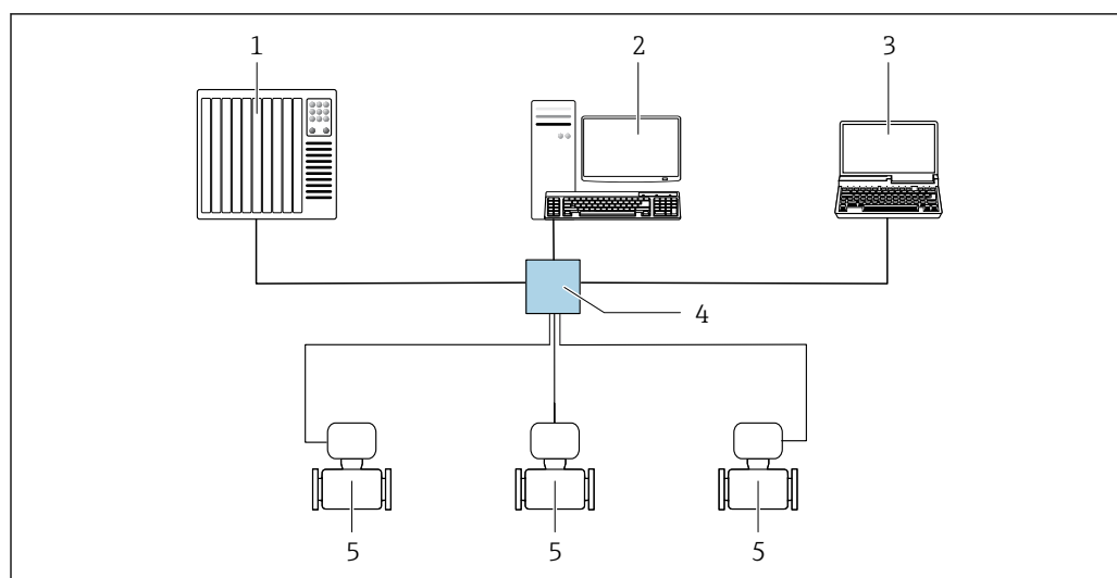
図 53 EtherNet/IP ネットワーク経由のリモート操作用オプション：スター型トポロジー
