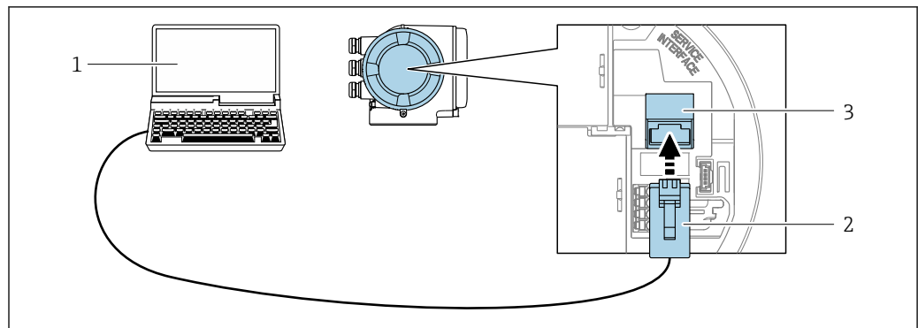
図 60 サービスインタフェース (CDI-RJ45) 経由の接続
