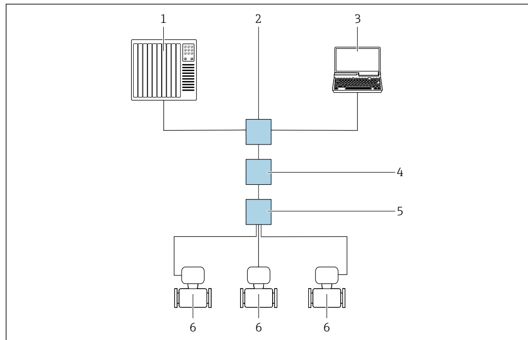
図 57 Modbus TCP over Ethernet-APL プロトコル経由のリモート操作オプション (アクティブ)
