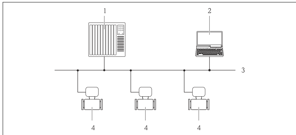
図 50 PROFIBUS DP ネットワークを介したリモート操作のオプション
