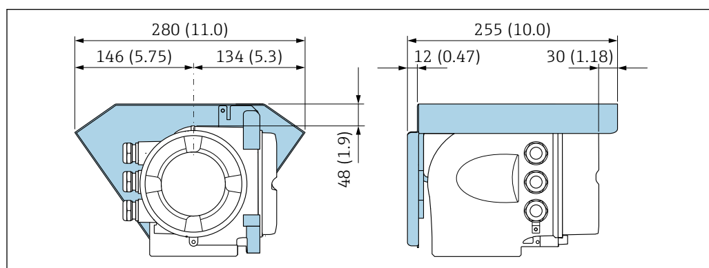
図 19 Proline 500 用の日除けカバー、単位 mm (in)
