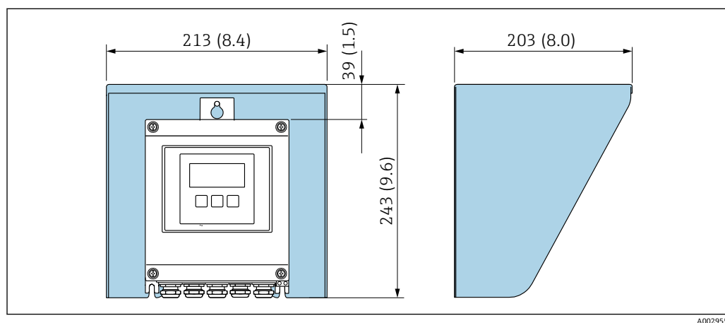
図 18 Proline 500 – デジタル用の日除けカバー、単位 mm (in)
