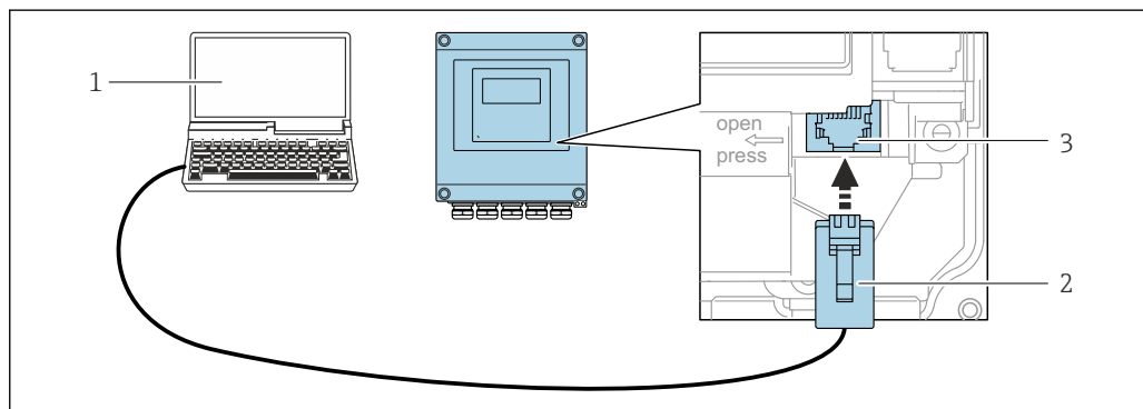
図 59 サービスインタフェース (CDI-RJ45) 経由の接続
