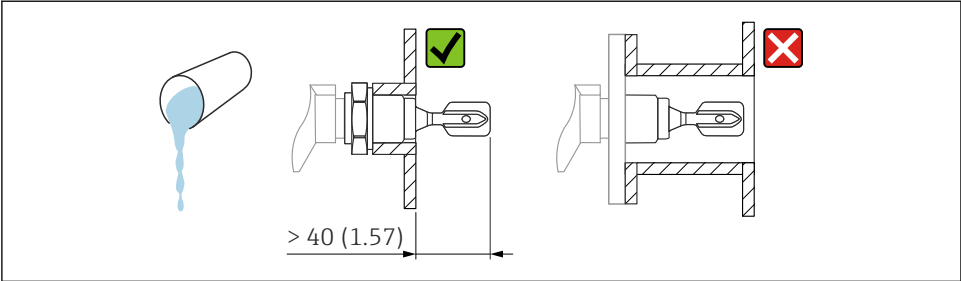
图 6 安装实例：测量高粘度液体介质。测量单位 mm (in)
