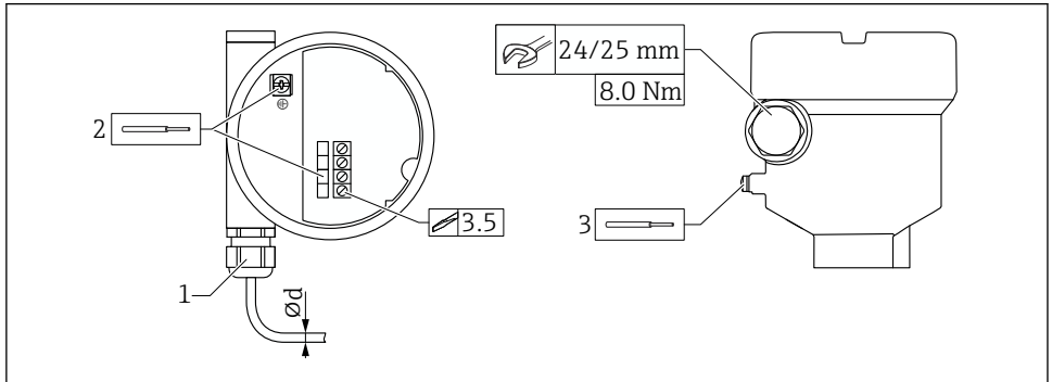
图 16 实例：缆塞（带电缆入口）和电子插件（带接线端子）
