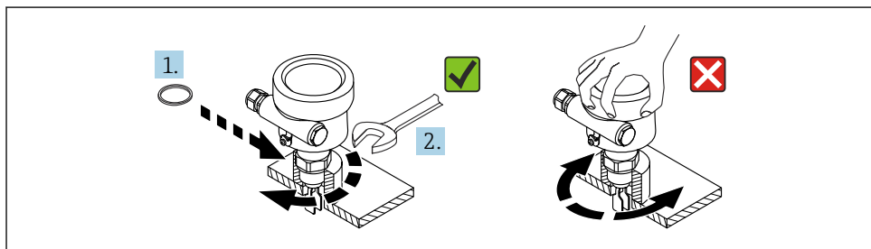
图 12 拧入设备
