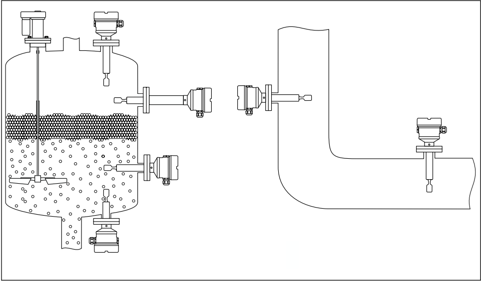
图 2 安装实例：安装在容器、罐体或管道中
