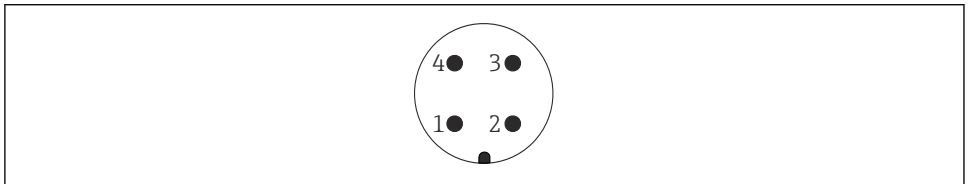
图 13 M12 插头的针脚分配
