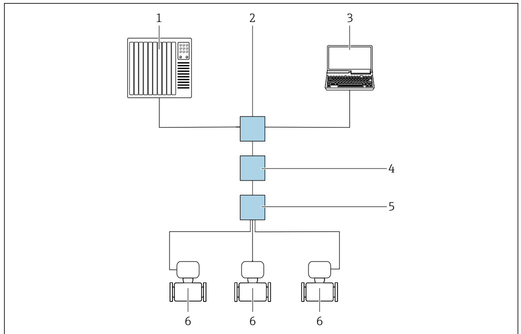
图 58 通过 Modbus TCP + Ethernet-APL 通信进行远程操作（有源信号）
