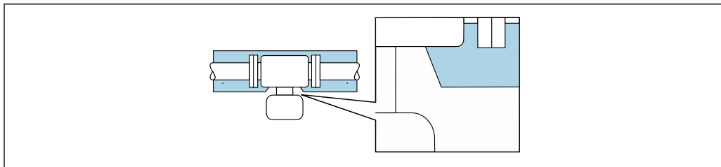
图 32 延长颈上无保温层覆盖
