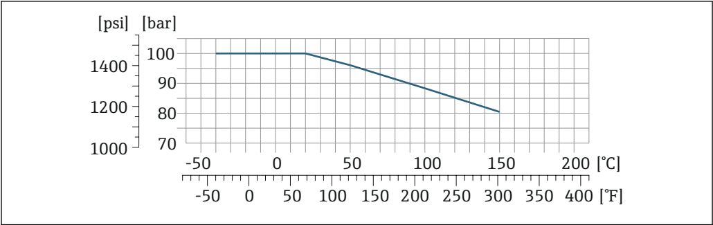
图 31 连接部件材质: 1.4404 (316/316L)
