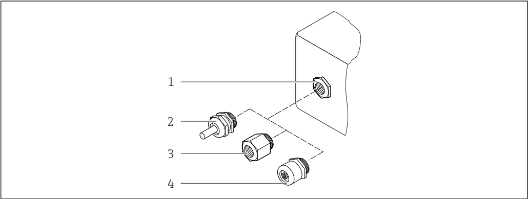
图 46 允许的电缆入口/缆塞
