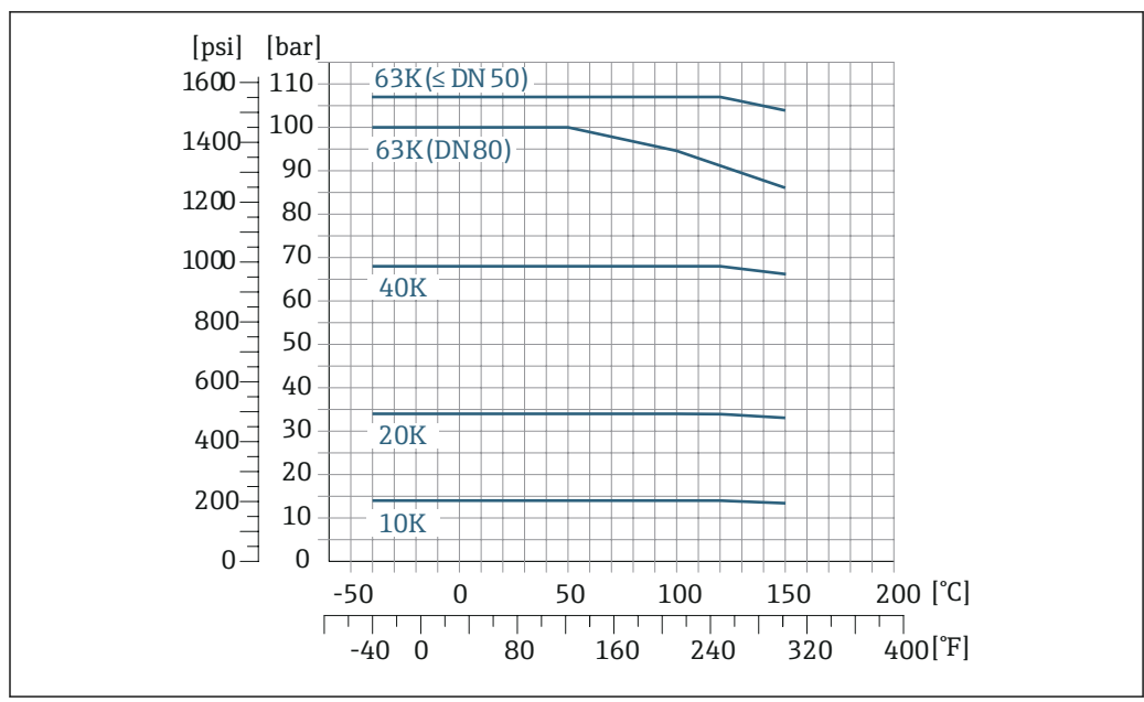
图 25 法兰材质: 1.4404 (F316/F316L)
