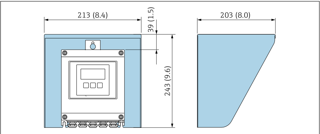
20 Proline 500（数字）变送器的防护罩；单位：mm (in)
