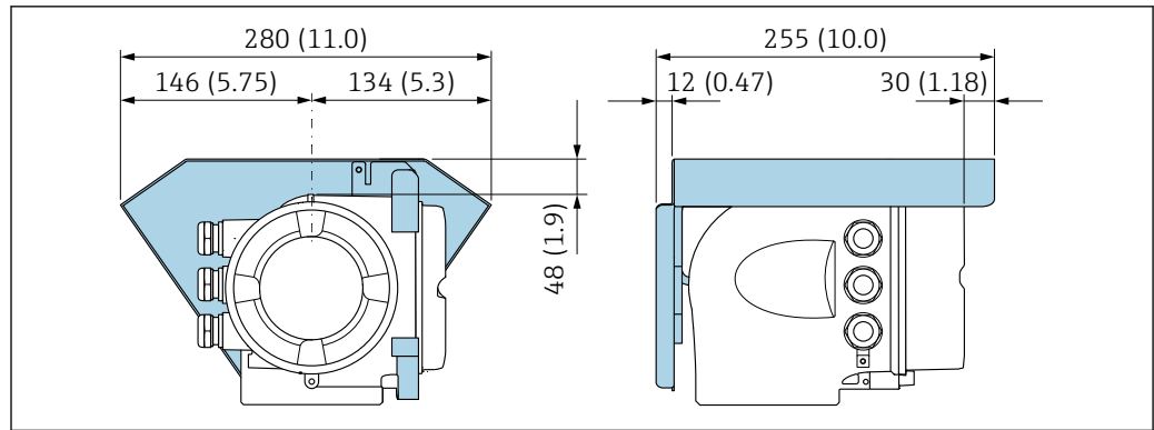
图 35 Proline 500 变送器的防护罩；单位：mm (in)
