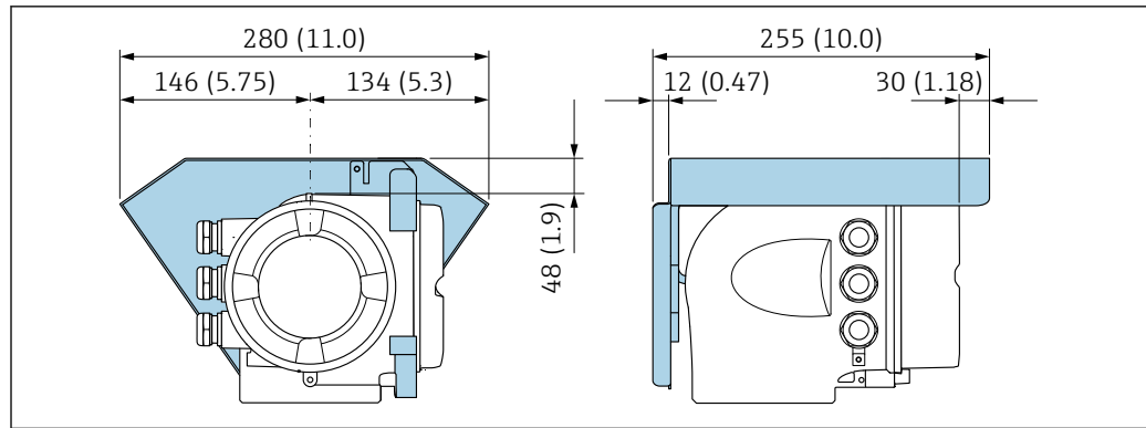
图 41 Proline 500 变送器的防护罩；单位：mm (in)
