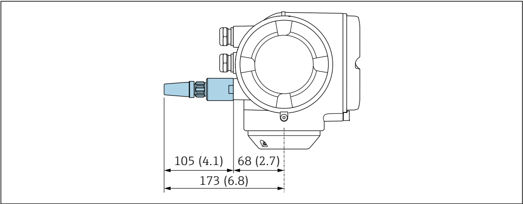
44 单位: mm (in)
