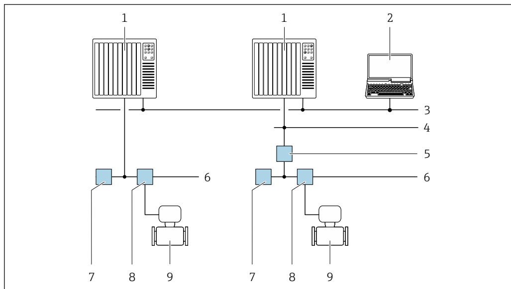
50 通过 FOUNDATION Fieldbus 网络进行远程操作
