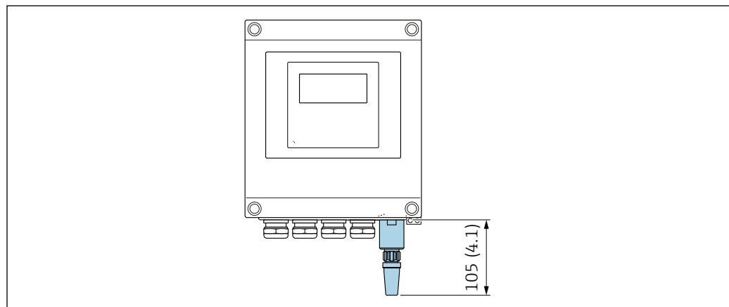
图 42 单位：mm (in)
