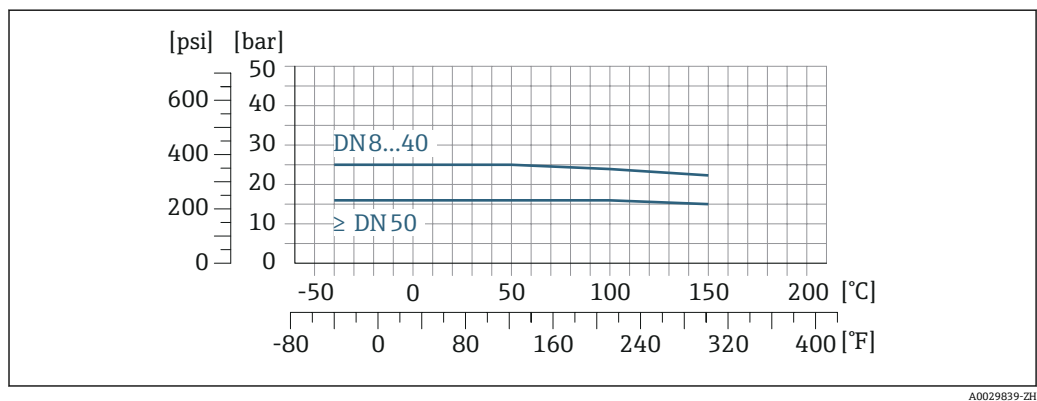
图 26 法兰材质: 1.4404 (316/316L)
