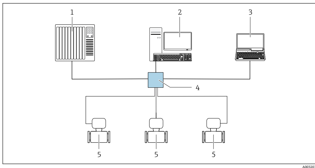
图 59 通过 Modbus TCP + Ethernet 进行远程操作 - 100 Mbit/s: 星形拓扑结构
