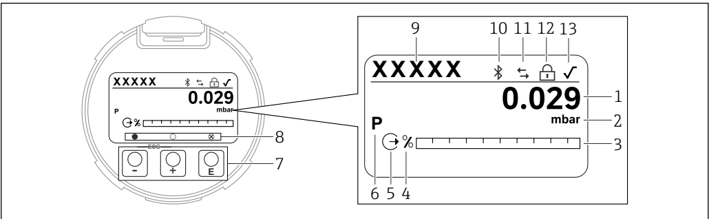
图 10 图形显示屏，带光敏键。
