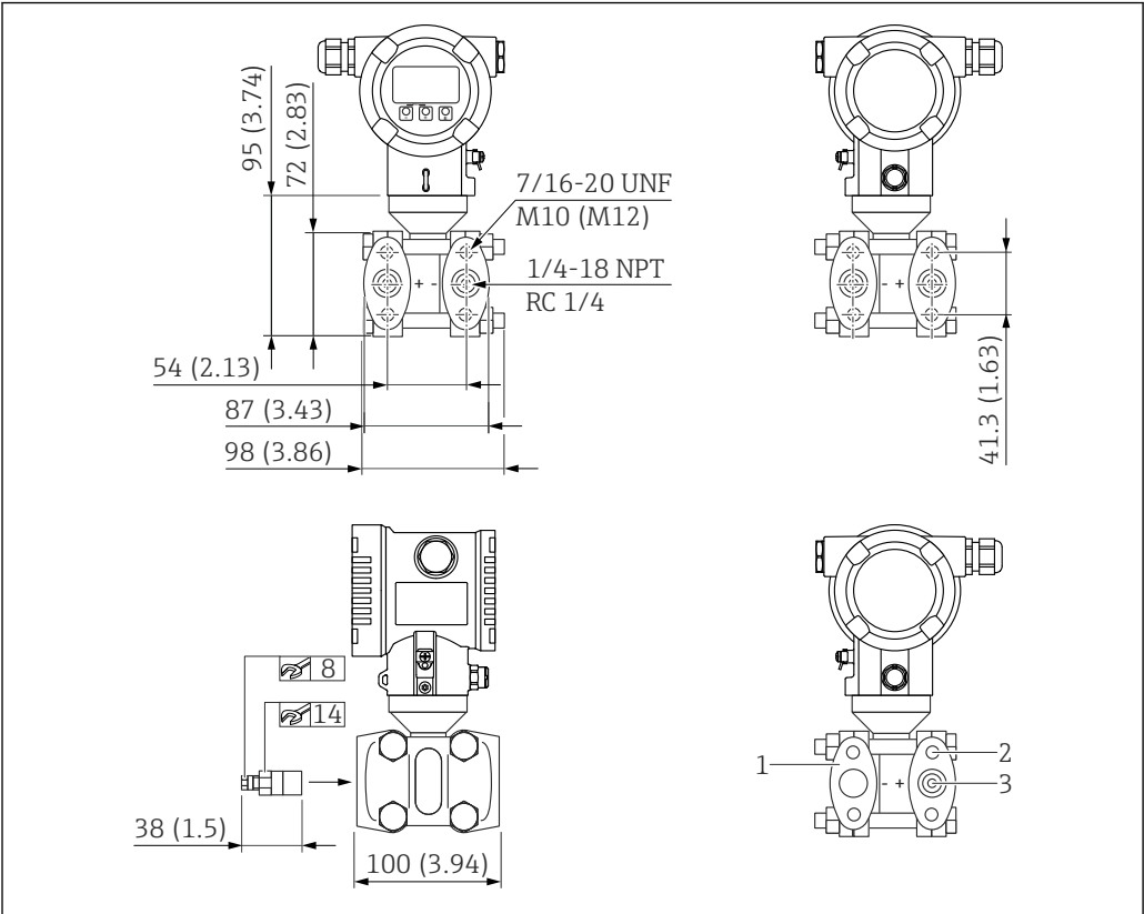
图 7 正视图、左视图、右视图。测量单位 mm (in)
