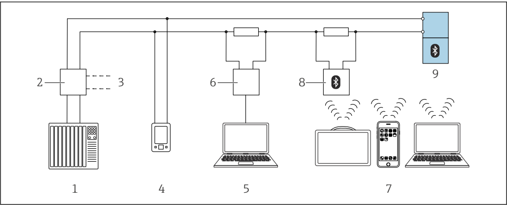
图 11 通过 HART 通信进行远程操作
