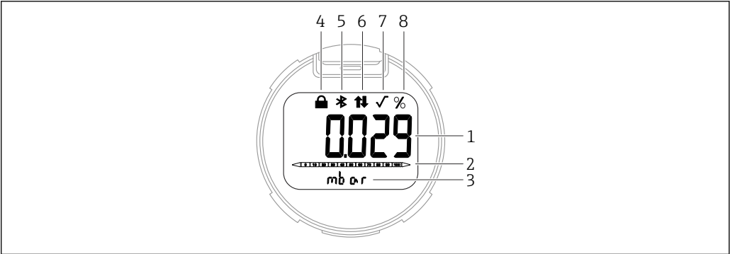
图 9 段码显示屏
