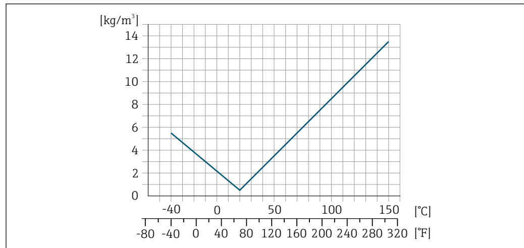
36 Калибровка по плотности на месте эксплуатации, в примере при +20 °C (+68 °F)
