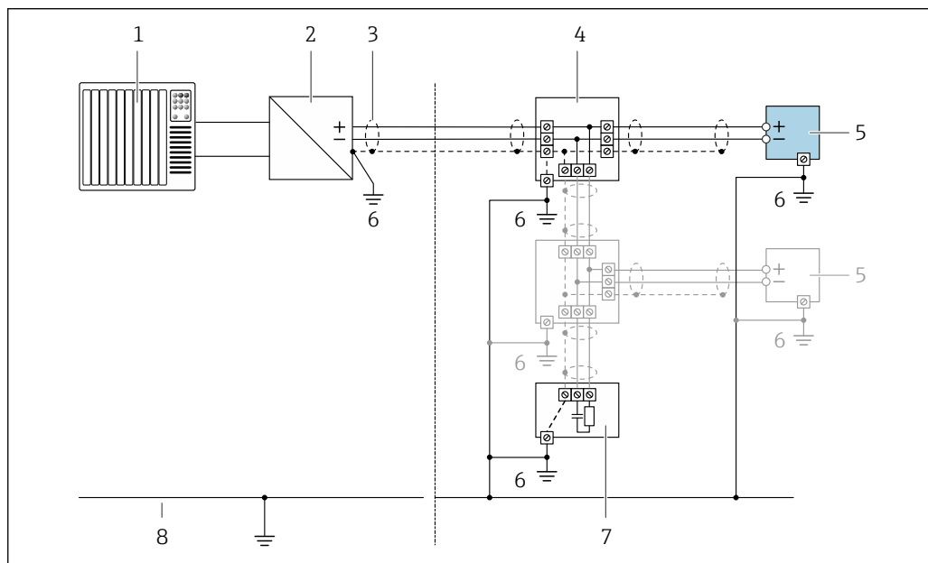
20 Пример подключения для интерфейса FOUNDATION Fieldbus
