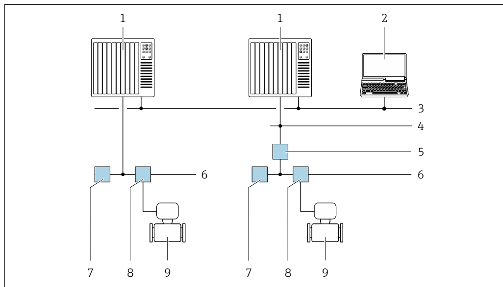
26 Варианты дистанционного управления по сети FOUNDATION Fieldbus
