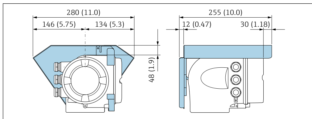
8 Ед. изм.: мм (дюймы)
